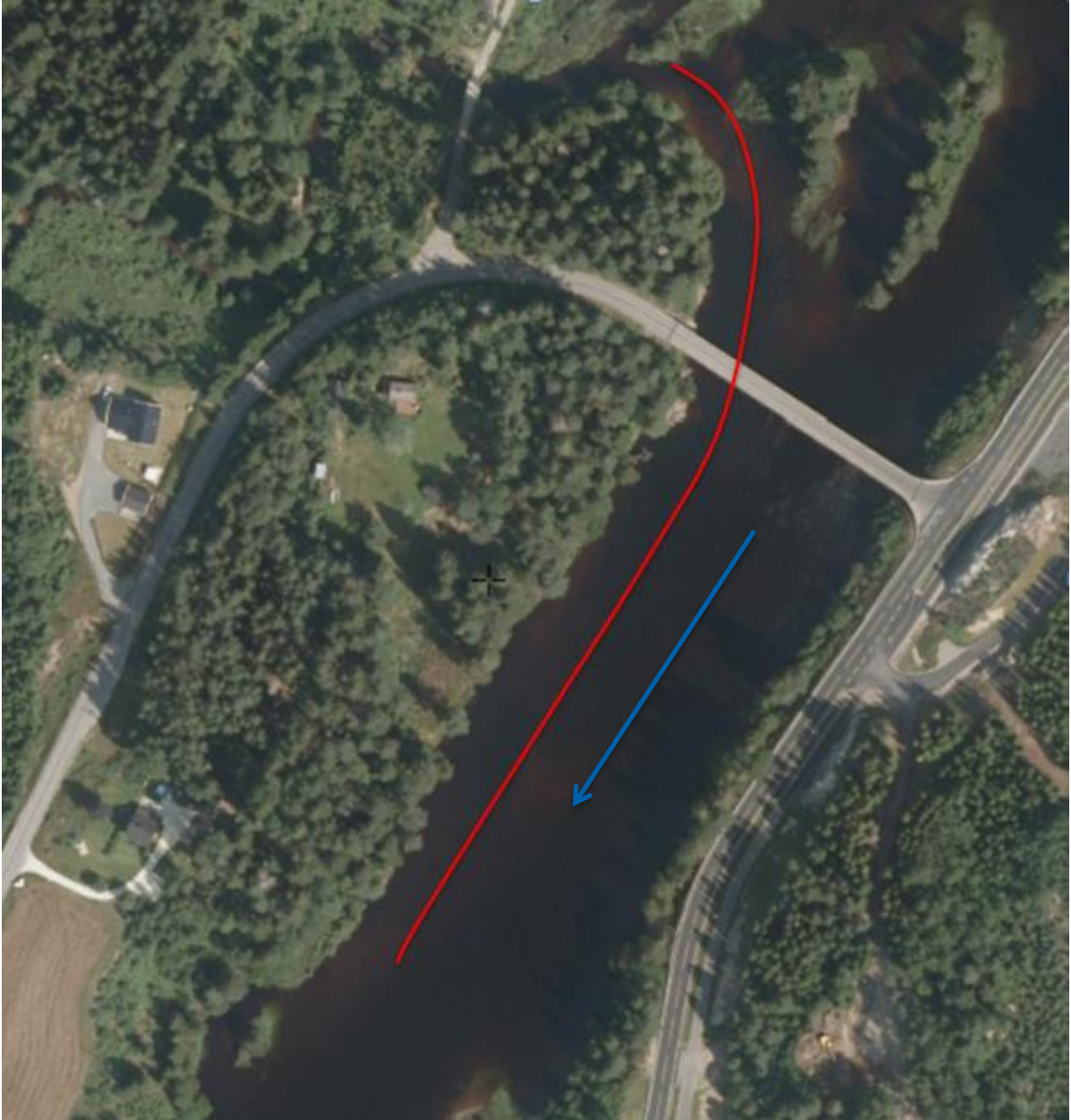
Figur 6. Flyfoto av områdene nedstrøms utløpet fra Monebekken. Denne delen av Tovdalselva renner nokså laminært slik at det er lite innblanding på tvers av elva. Brunfargen er fargen på bunnsubstratet som består av stein og grus. Fotoet viser derfor hvor grunn elva er i dette området. Det er uvisst hvor langt nedover i elva fisk er påvirket av giftige overgangsformer av aluminium på grunn av surt vann fra Monebekken. Kilde Norkart AS.
