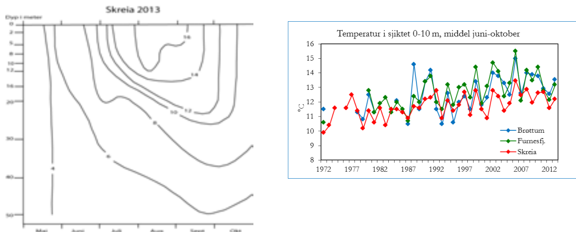
Figur 3. Isotermidiagram for stasjon Skreia i 2013 (til venstre) og tidsutviklingen i middeltemperaturen i de øvre, varme vannlag (0-10 m) i perioden juni-oktober ved stasjonene Brøttum, Furnesfjorden og Skreia (til høyre).
