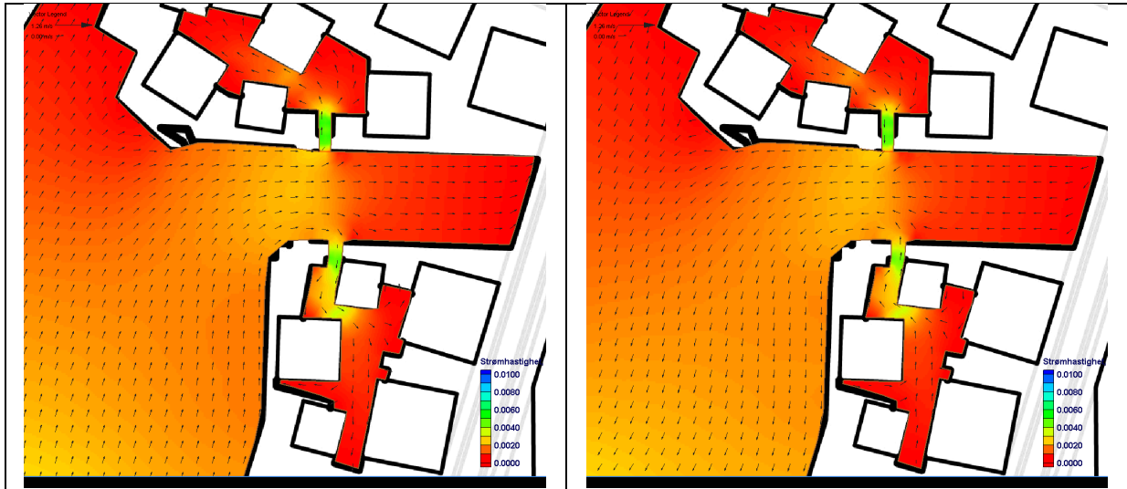
Figur 10. Scenario 3: Simulering av vannsirkulasjon i 0-1,5 m dyp i bassengene ved middels tidevannsvariasjon og stor vannføring ( 40 \text{ m}^3/\text{s} ) i Akerselva. Venstre figur: innstrømmende tidevann. Høyre figur: utstrømmende tidevann. Nederst til høyre i hver figur: skala for strømhastighet går fra 0 (rød) til 0,01 (blå) m/s.
