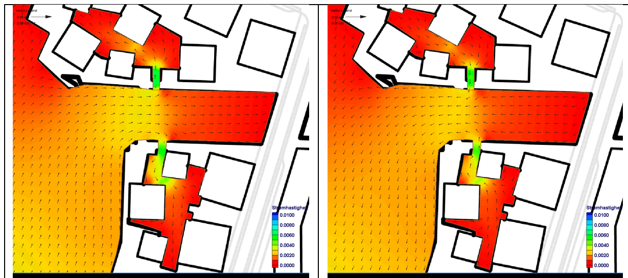
Figur 12. Scenario 5: Simulering av vannsirkulasjon i 0-1,5 m dyp i bassengene ved stor tidevannsvariasjon og vannføring 17,5 m 3 /s i Akerselva. Venstre figur: innstrømmende tidevann. Høyre figur: utstrømmende tidevann. Nederst til høyre i hver figur: skala for strømhastighet går fra 0 (rød) til 0,01 (blå) m/s.
