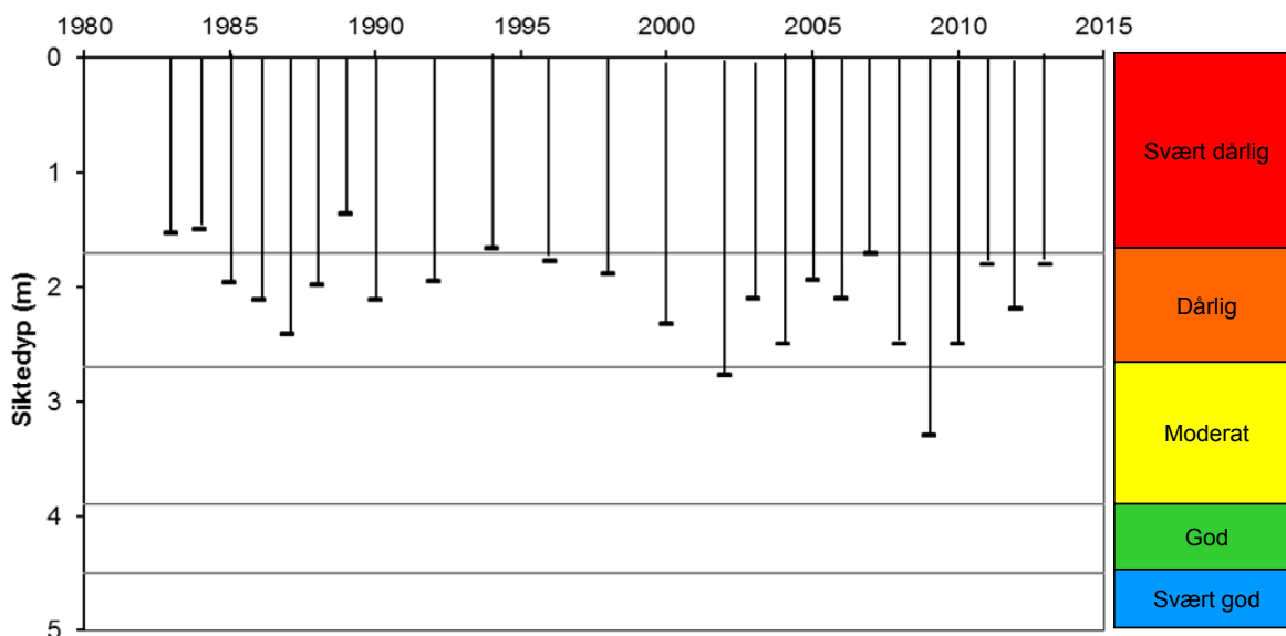
Figur 24. Gjennomsnittlig siktedyp (meter) i Kolbotnvannet for årene 1983-2013. Figuren viser middelverdien av siktedyp for hvert år, samt grensene mellom de ulike økologiske tilstandsklassene i klassifiseringssystemet til vannforskriften.
