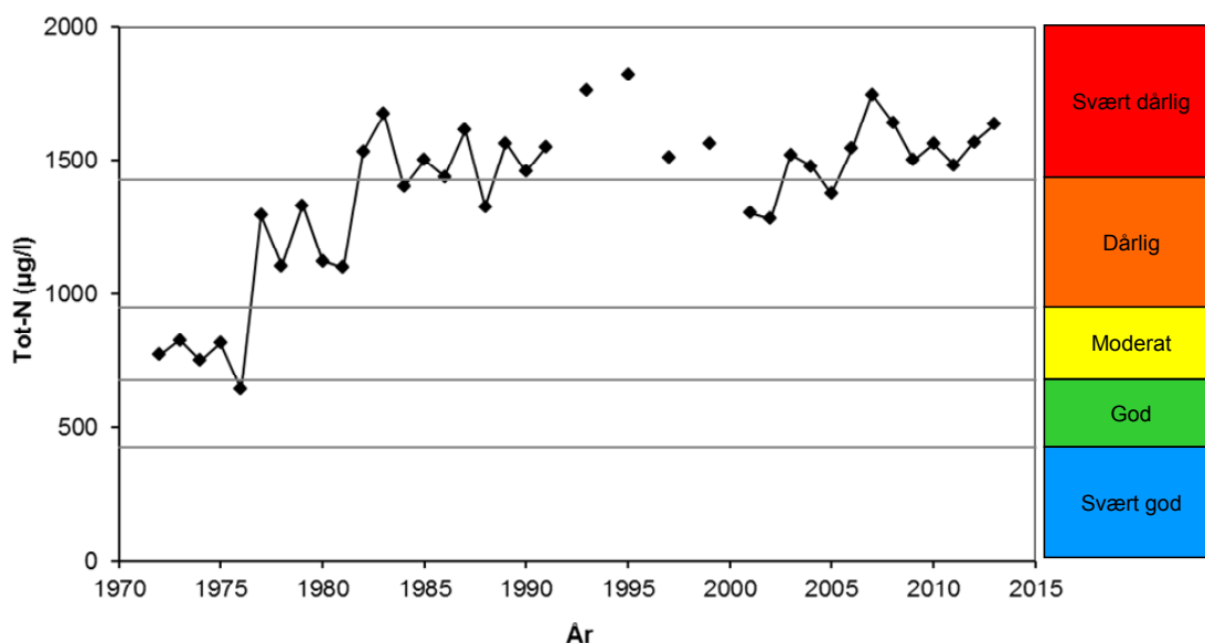
Figur 12 Nitrogenkonsentrasjon i Gjørsjøen 0-10 meters dyp for perioden 1971-2013. Figuren viser middelverdien av totalt nitrogen for hvert år, samt grensene mellom de ulike økologiske tilstandsklassene i klassifiseringssystemet til vanddirektivet.
