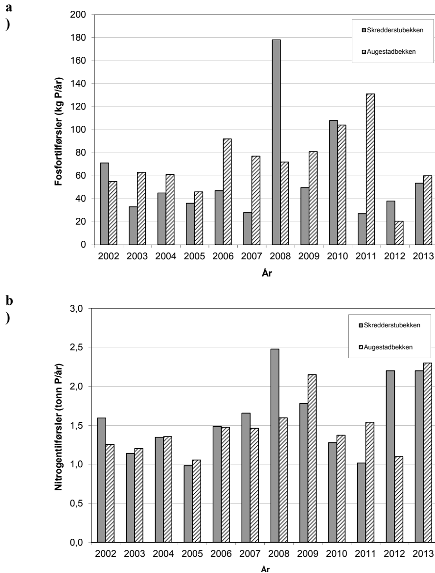
Figur 21. Tilførsler av a) fosfor og b) nitrogen til Kolbotnvannet fra Augestad- og Skredderstubekken i 2002-2013.
