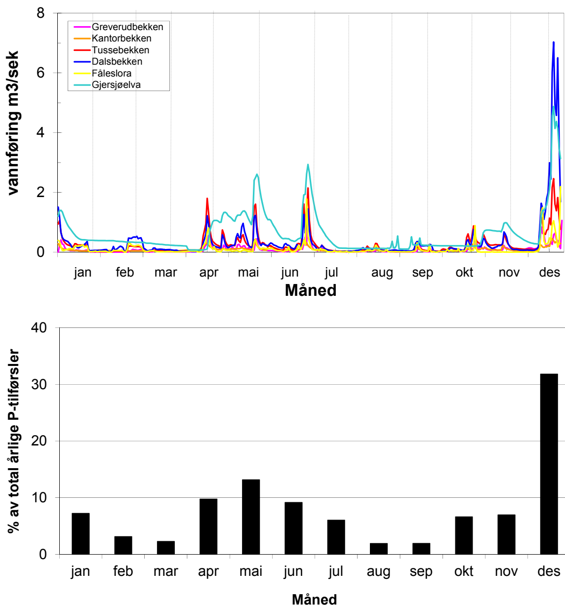
Figur 2. Vannføring (øverst) og fordeling av fosfortilførsler (nederst) fra Gjersjøbekkene i 2013. Datoer for prøvetagning i bekkene er vist med stiplede, vertikale linjer i øverste figur.
