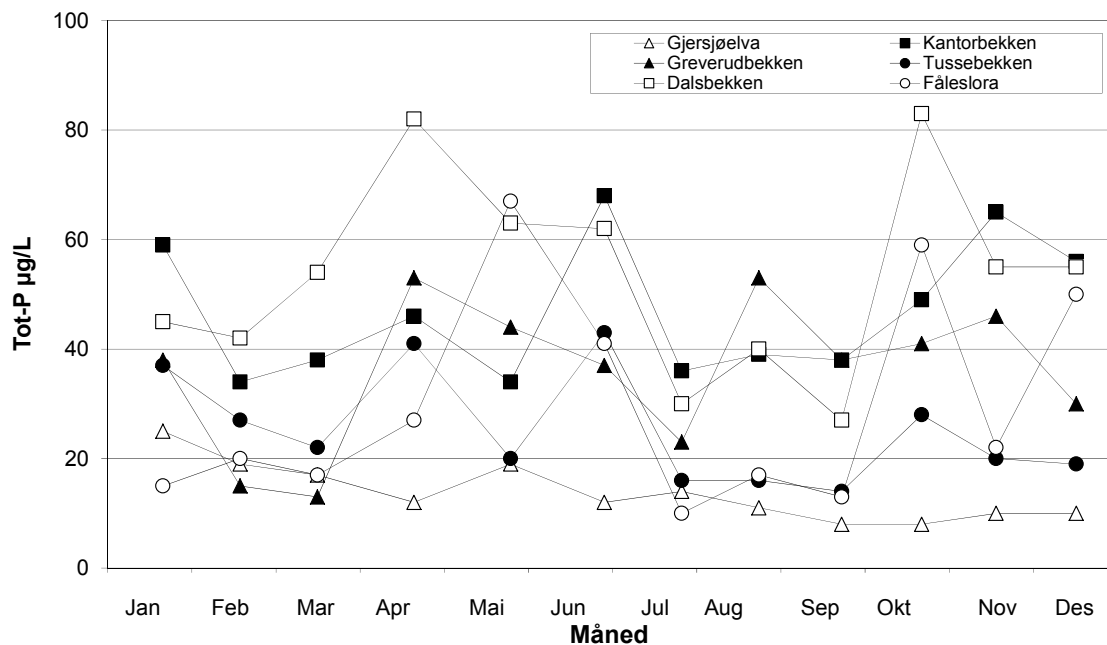
Figur 1. Målte fosforkonsentrasjoner i Gjersjøbekkene i 2013.
