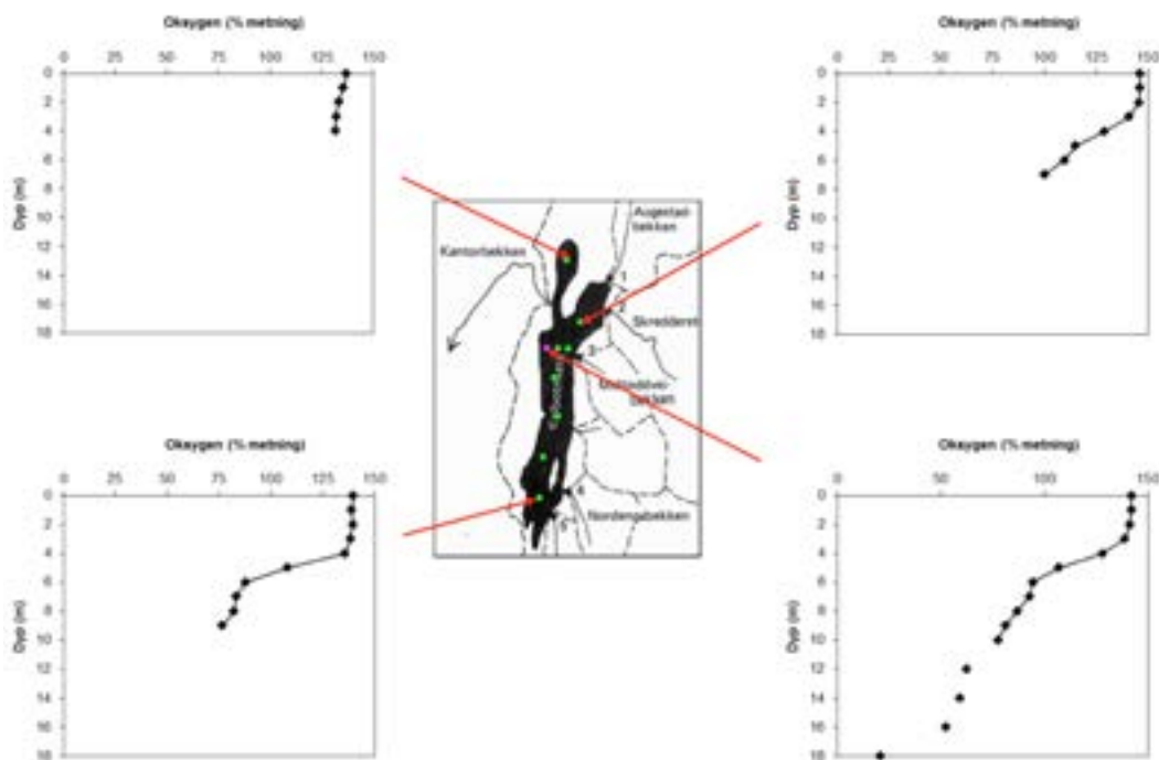
Figur 9. Oksygenprofiler på flere stasjoner i Kolbotnvannet den 02.07.2013.
