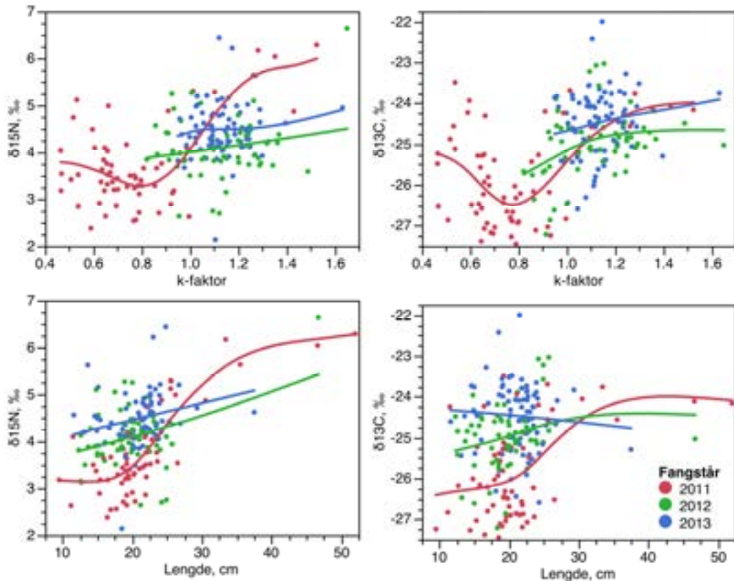
Figur 22. Stabile N- og C-isotoper som funksjon av kondisjonsfaktor ( k -faktor) og lengde hos ørret fra Ringedalsvatnet. Røde punkter er fra juni og blå punkter er data fra september (2011). Kurvene er laget med kurveglattingsfunksjoner (smoothing splines).
