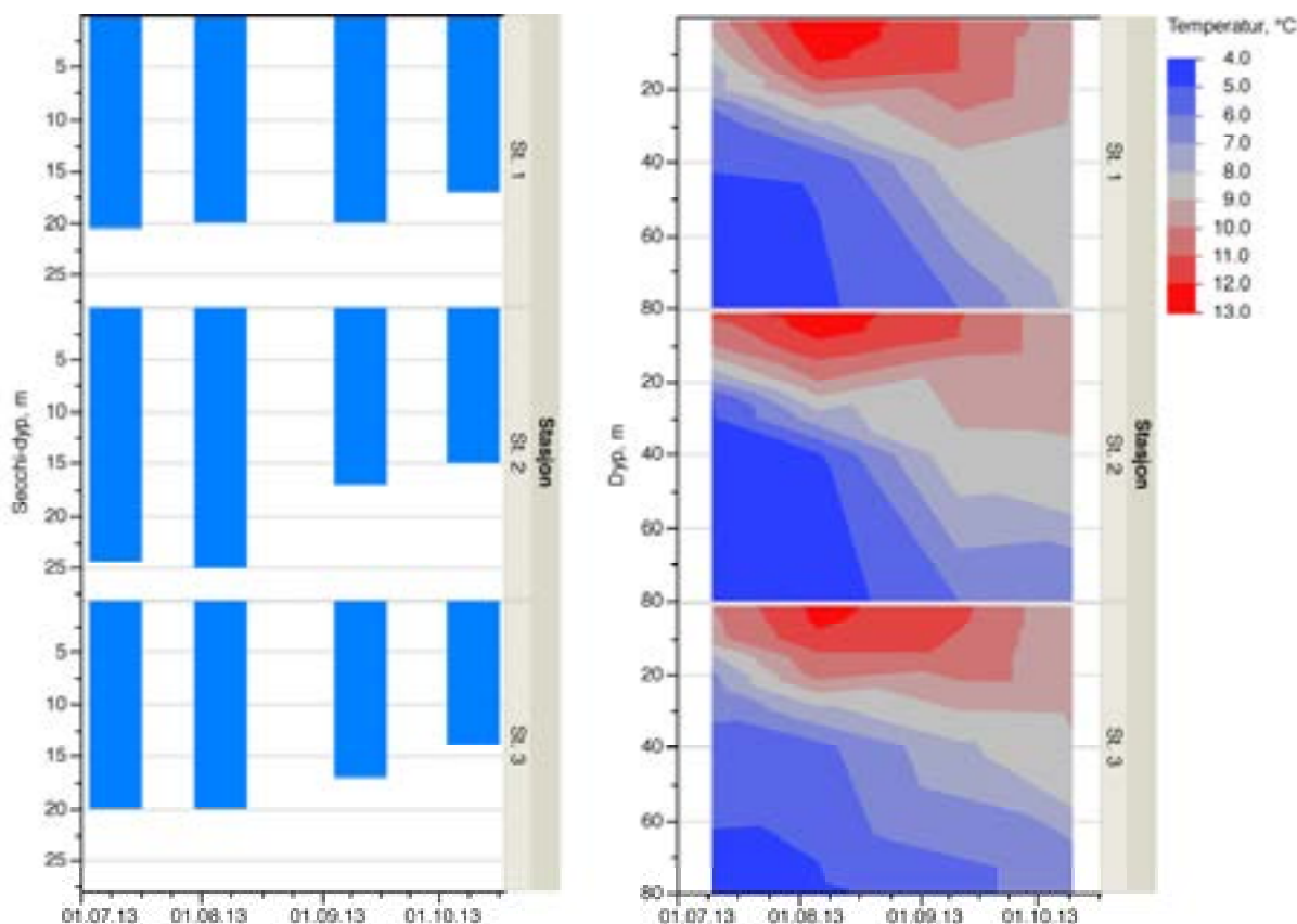
Figur 7. Siktedyp (Secchi-dyp, venstre figur) og temperatur-isotermer (høyre figur) ved tre stasjoner i Ringedalsvatn for perioden 10. juni – 10. oktober, 2013.
