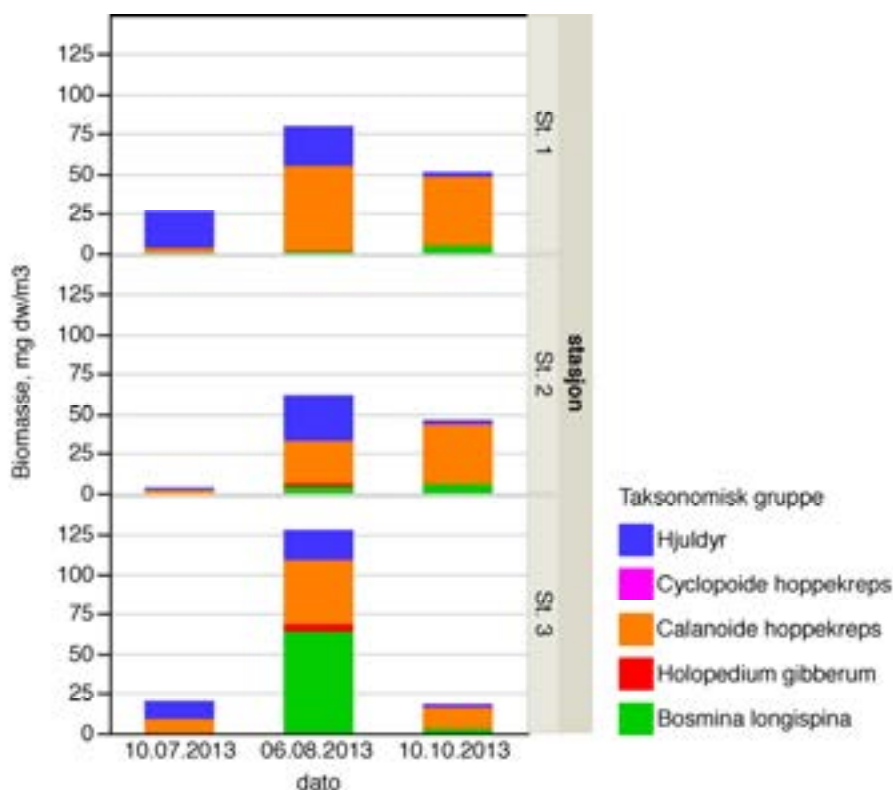
Figur 12. Utviklingen i zooplanktonsamfunnets ulike hovedgruppers biomasse (mg/m 3 , tørrvekt) i sjiktet 0-10 m ved tre stasjoner i Ringedalsvann i perioden juli–oktober 2013.
