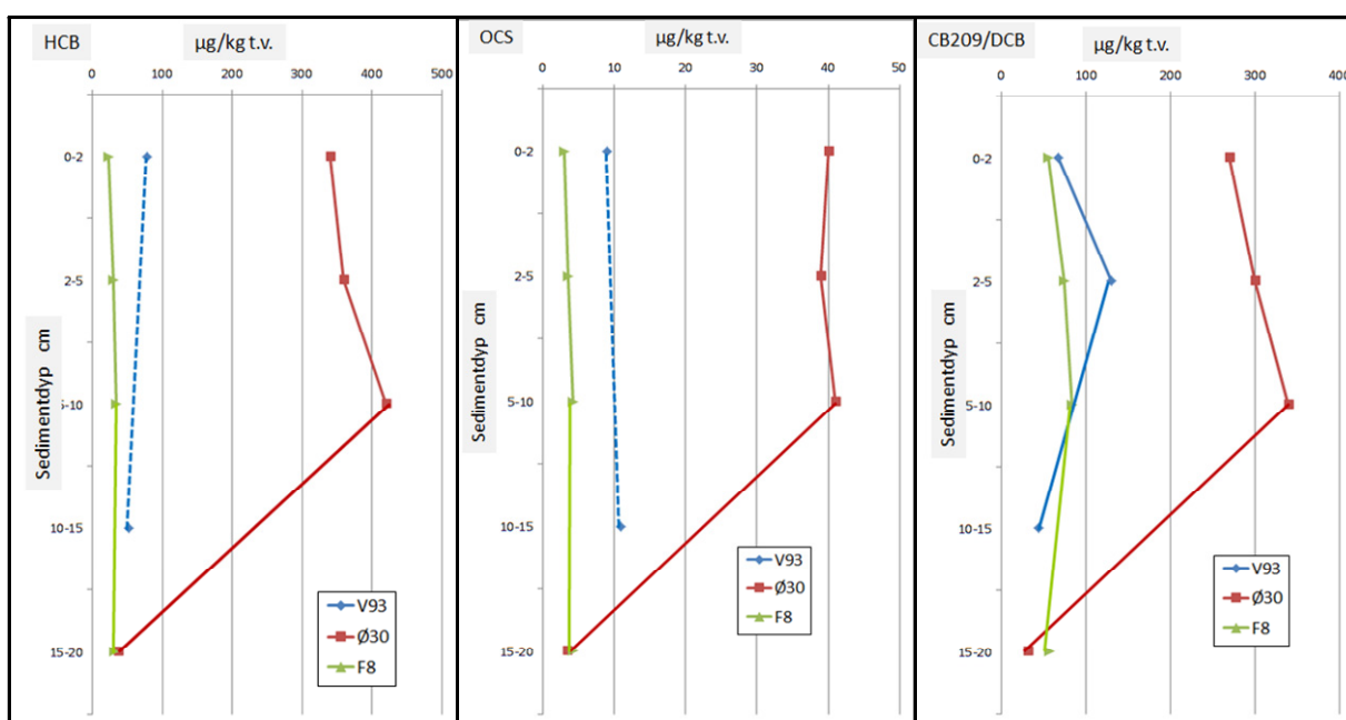
Figur 5. Vertikalfordeling (µg/kg t.v.) av HCB, OCS og DCB (PCB209) i sedimentet på to stasjoner i Frierfjorden (Ø30 og V93) og en stasjon i Langesundsfjorden (F8). NB ulik skala på horisontalaksen. Klasse V: > 50 µg/kg t.v.
