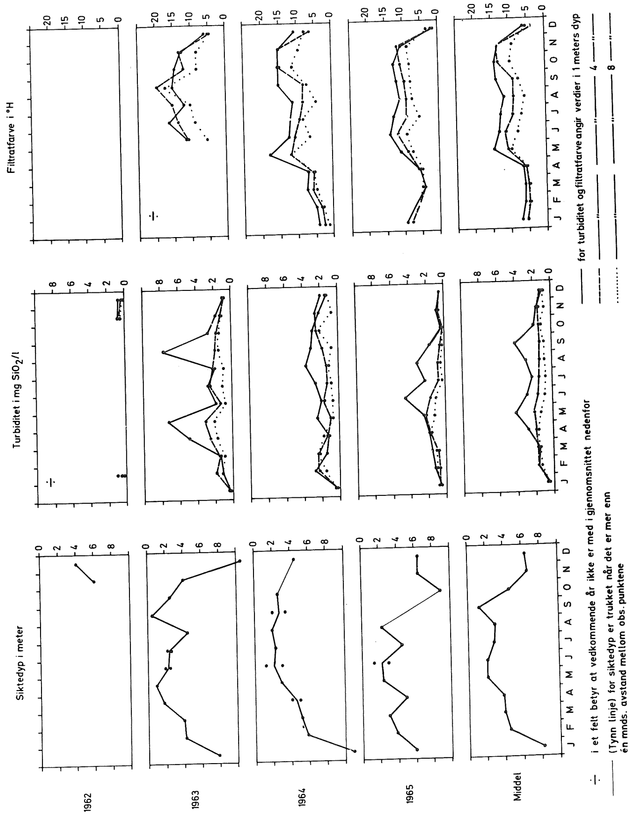
Månedsvariasjoner i siktedyp, turbiditet og filtratfarve ved stasjon Bn 1
