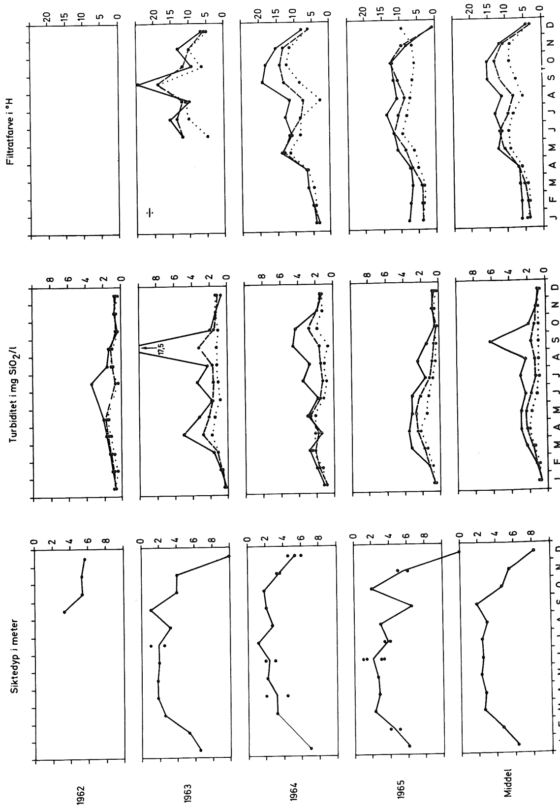
Fig.3b Månedsvariasjoner i siktedyp, turbiditet og filtratfarve ved stasjon CQ 1
