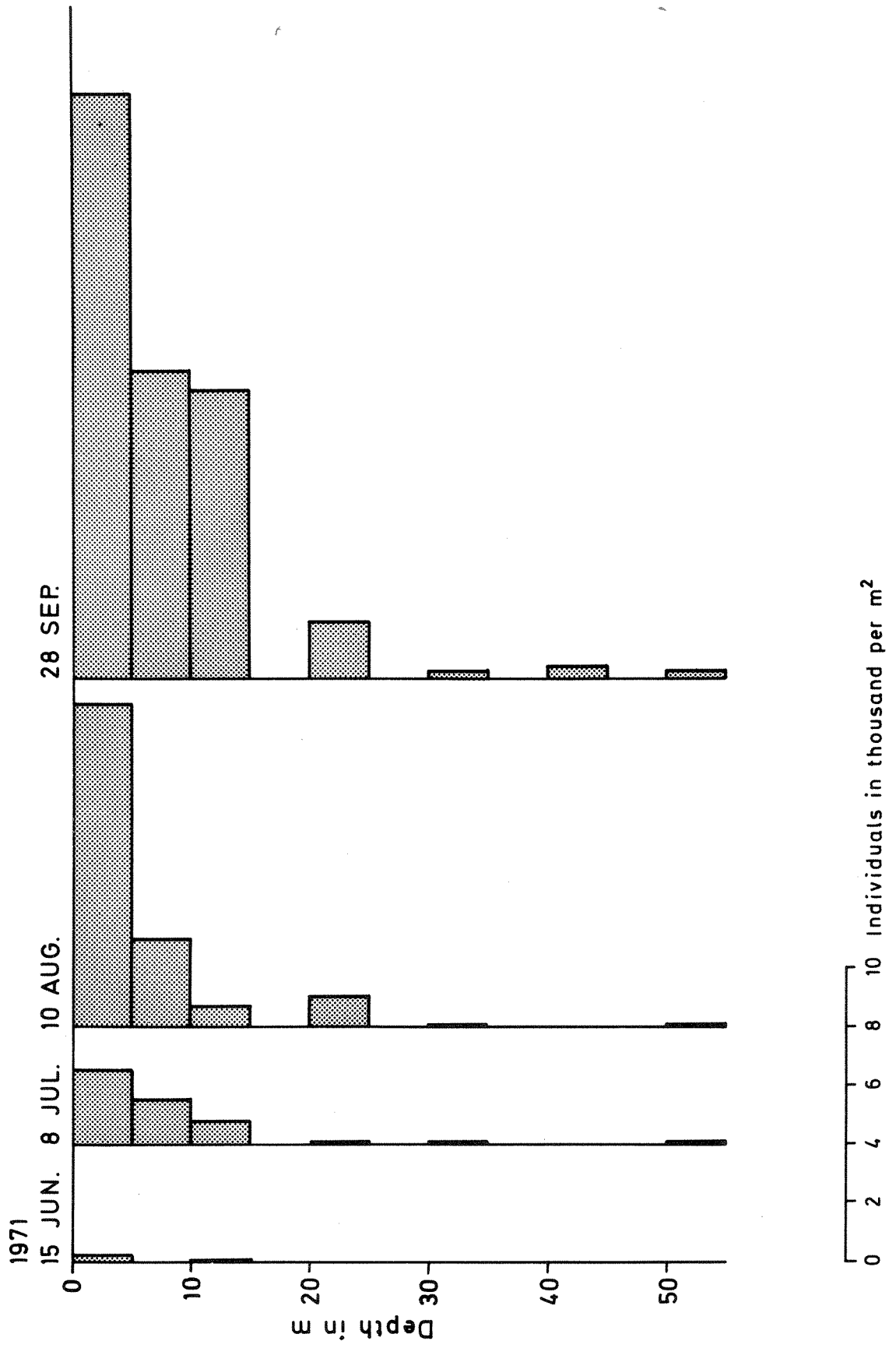
Figur 2. Vertikalfordeling av Daphnia galeata (krepsdyr) i Holsfjorden 15. juni, 8. juli, 10. august, 28. september 1971.
