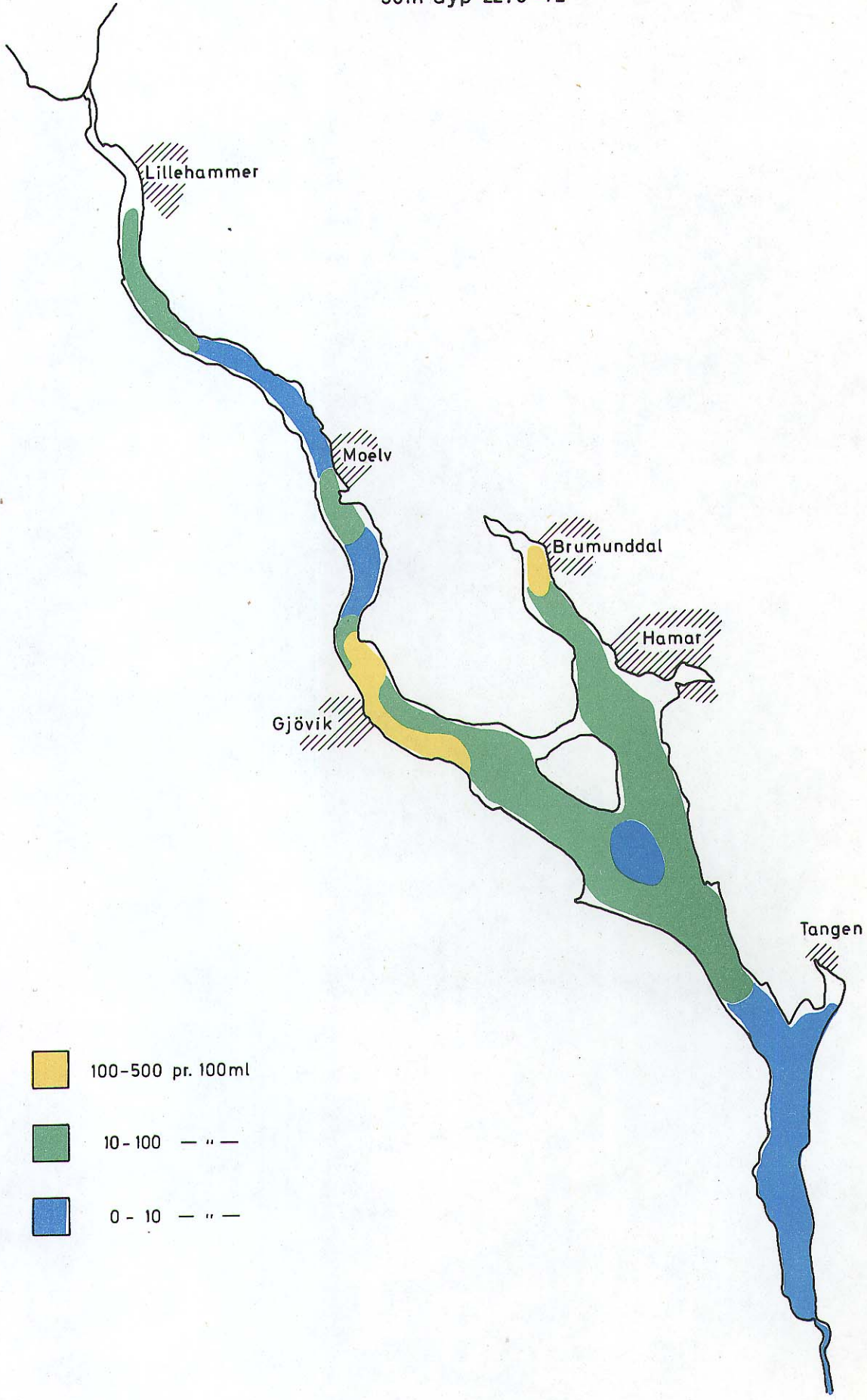
Fig. 31 Situasjonsbilde av coliforme bakterier (37°) i Mjøsa på 30m dyp 22/8 -72
