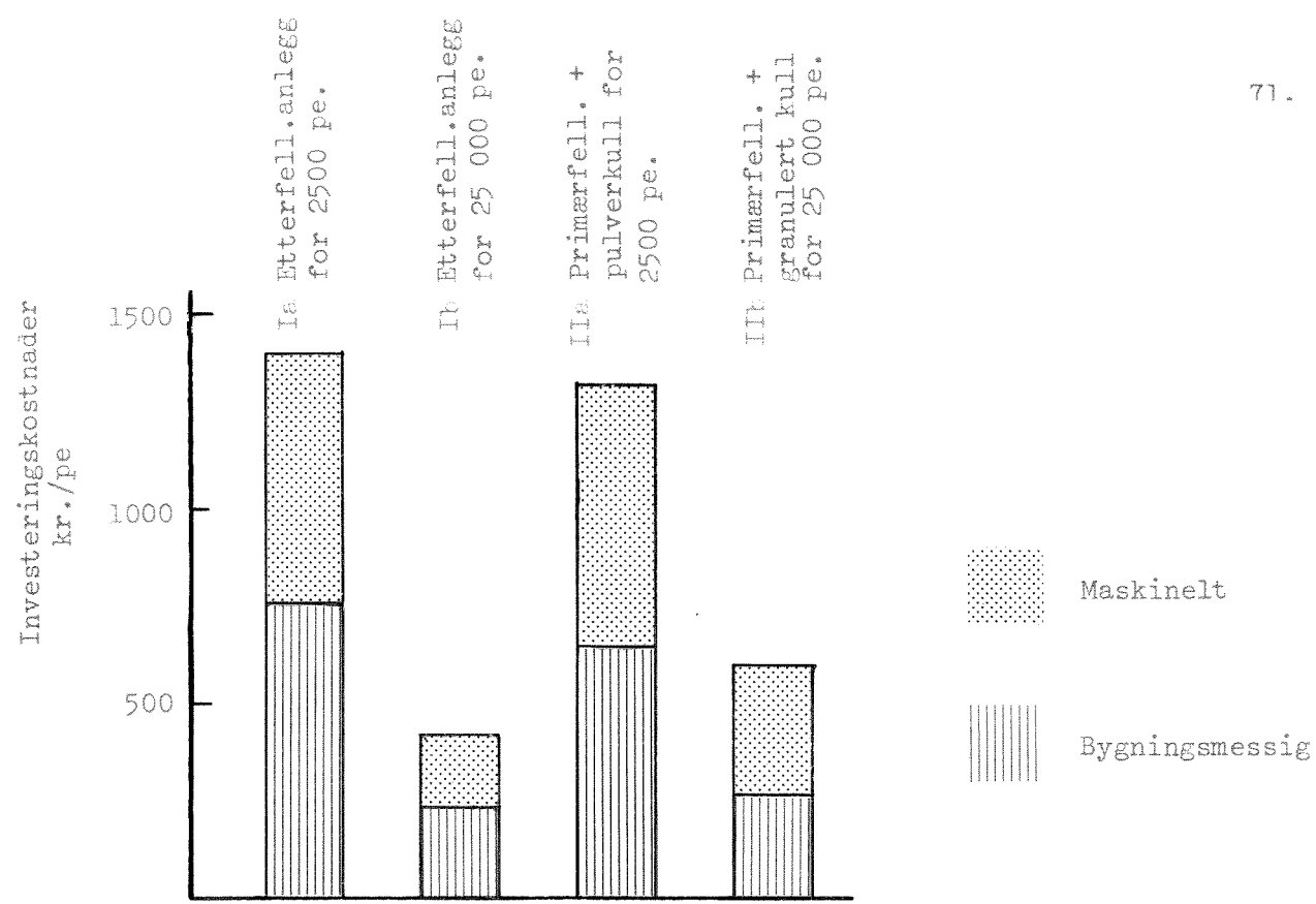
Fig.31 Grafisk fremstilling av spesifikke investeringskostnader (kr./pe) for de fire alternativer.
