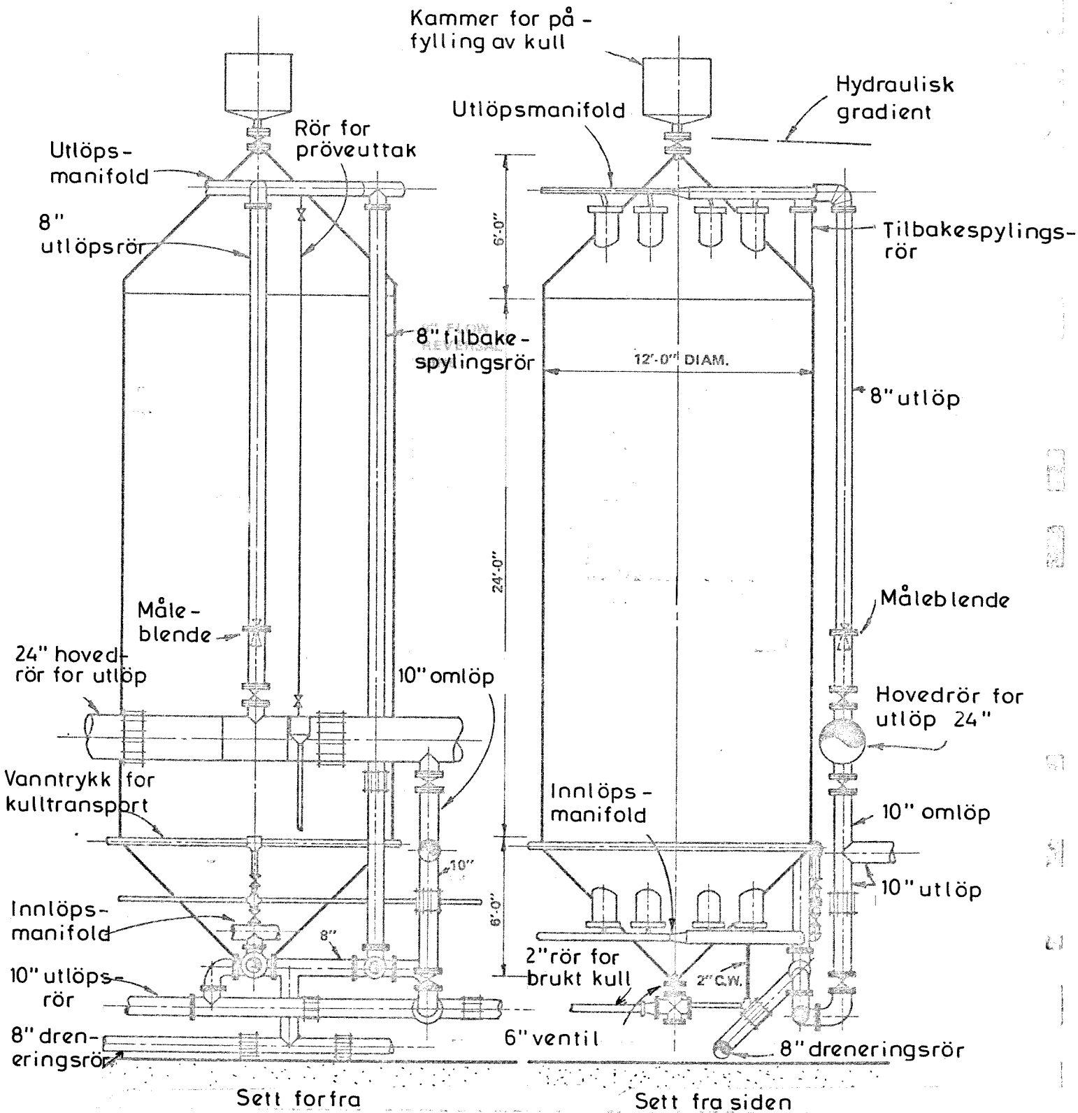
Fig. 9 Oppstrøms kolonne med vann og kull i motstrøm Orange county, California (EPA's design manual for activated carbon, 1973)
