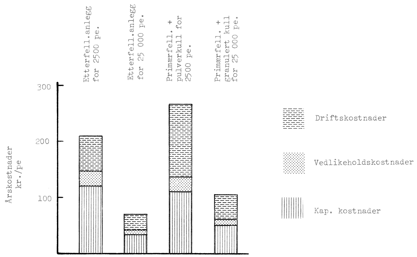
Fig.32 Grafisk fremstilling av spesifikke årskostnader (kr./pe) for de fire alternativer.
