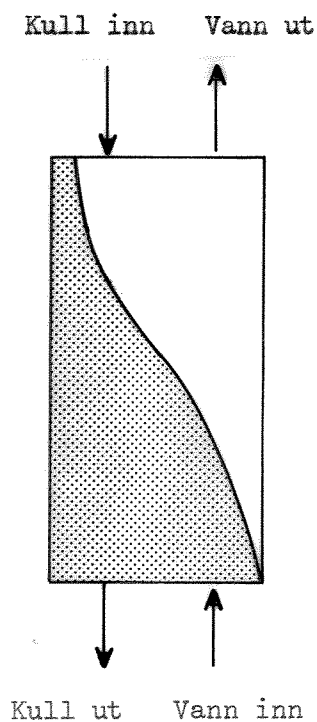
Fig.17 Prinsippskisse av konsentrasjonsprofilen i en kontinuerlig drevet kolonne med vann og kull i motstrøm.
