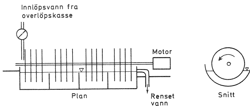
Fig.8 Prinsippkisse av kontaktvalse
