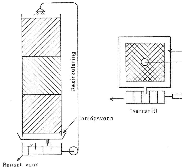
Fig.9 Prinsippkisse av rislefilter
