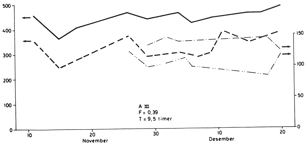
Fig.13 REDUKSJON AV KJEMISK OKSYGENFORBRUK OG ORGANISK KARBON FORSÖKSSERIE NR.4
