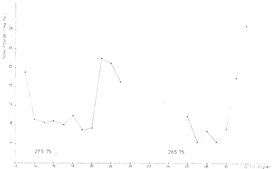
Fig 6 TOTAL FOSFOR I KONTORAVLOPSVANN FRA NORVEGIAS BYGG I BÆRUM
