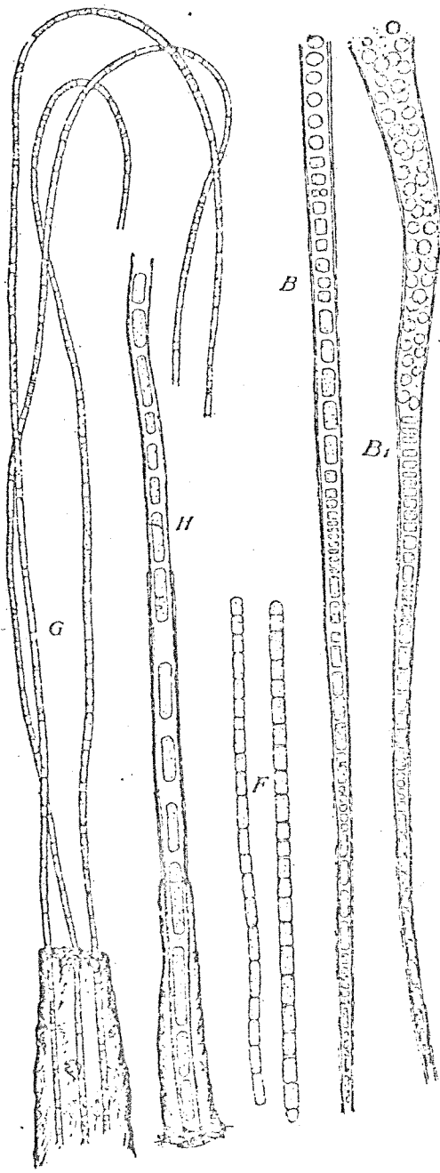
Abb. 35: Crenothrix polyspora .
