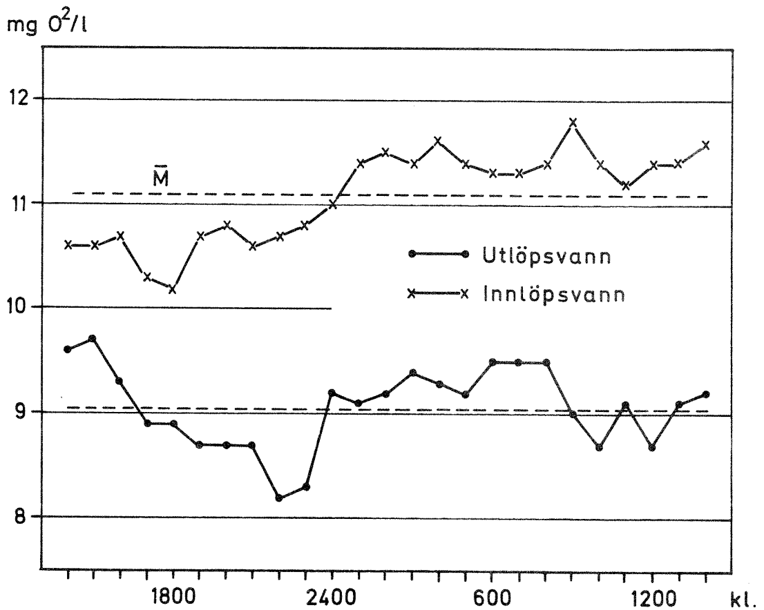
Fig.3 Variasjon av oksygeninnhold i innlöps- og utløpsvann
