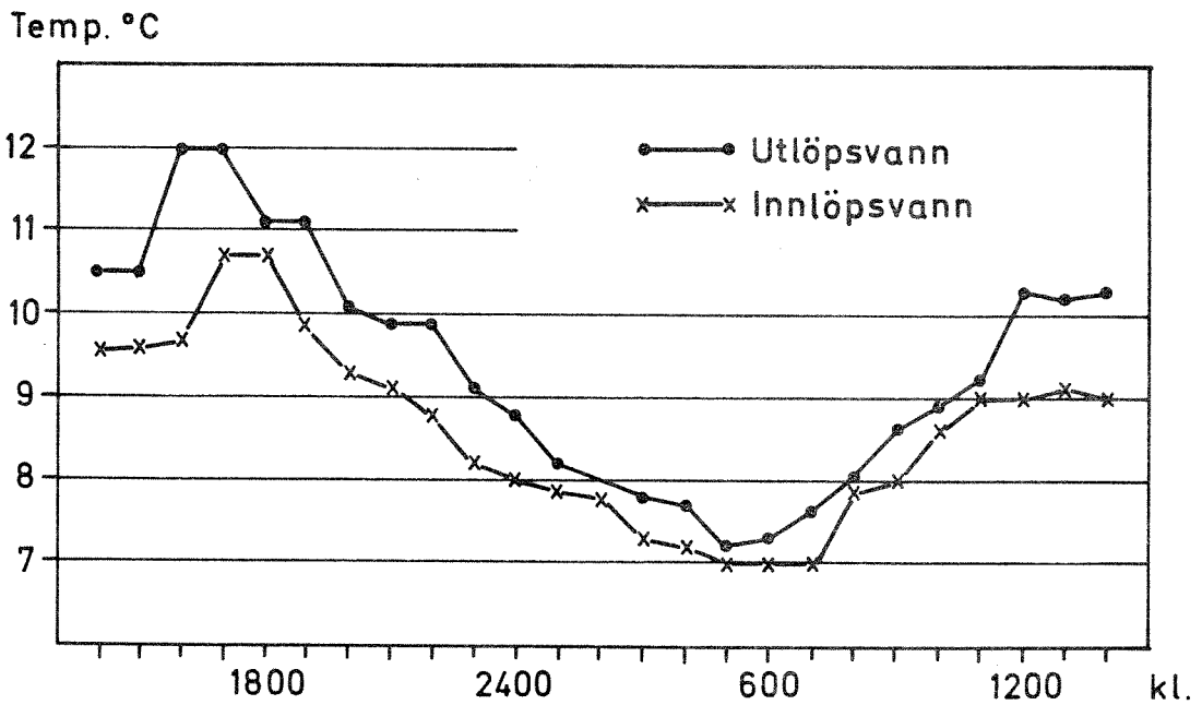
Fig.2 Temperaturvariasjoner i innlöps- og utløpsvann
