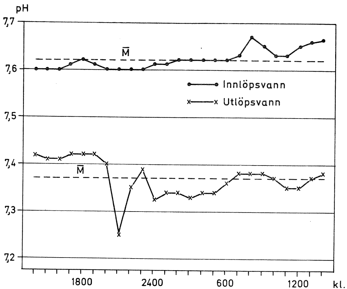
Fig.4 pH-variasjoner i innlöps- og utlöpsvann
