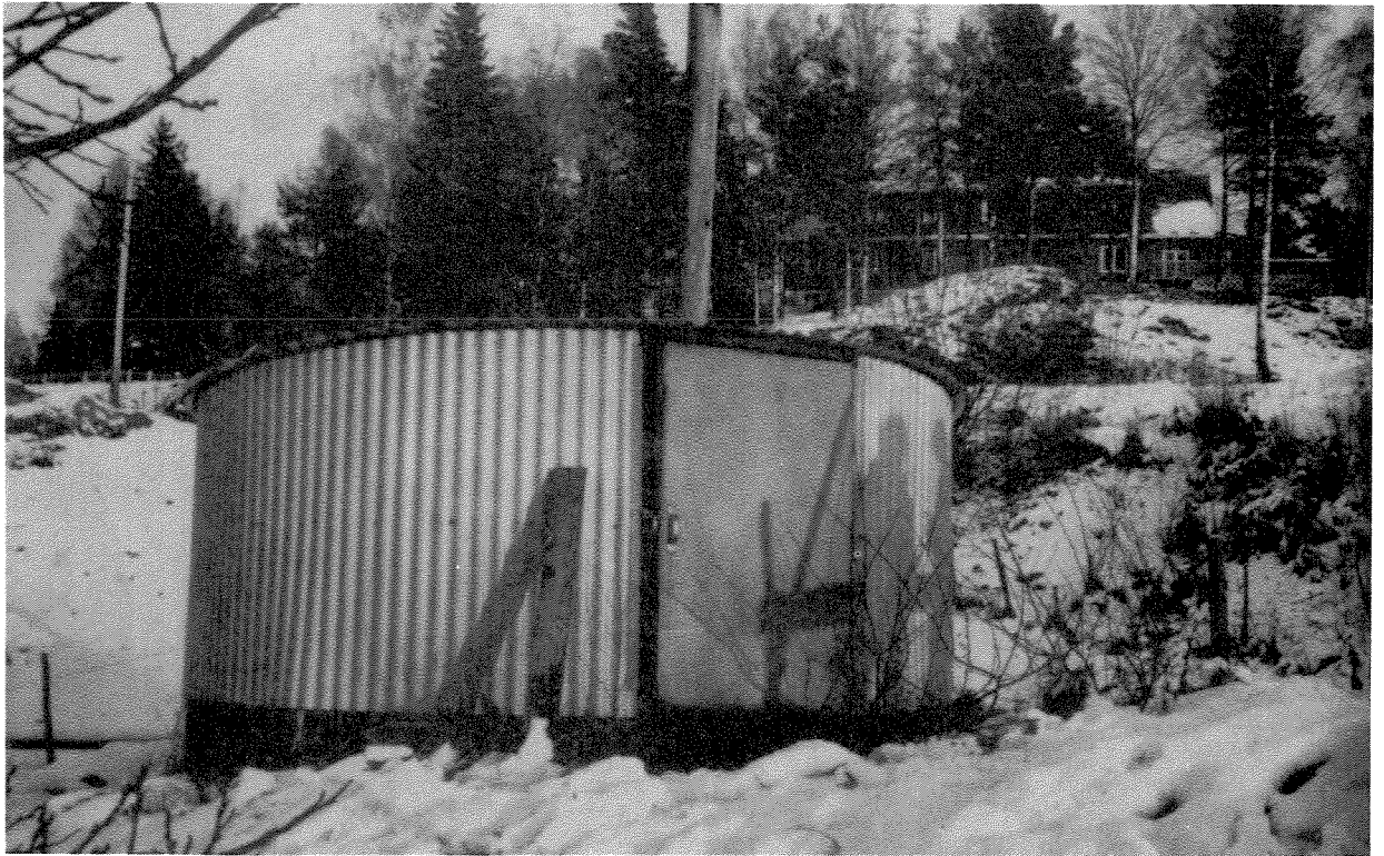
Enebakk sykestue's renseanlegg.
