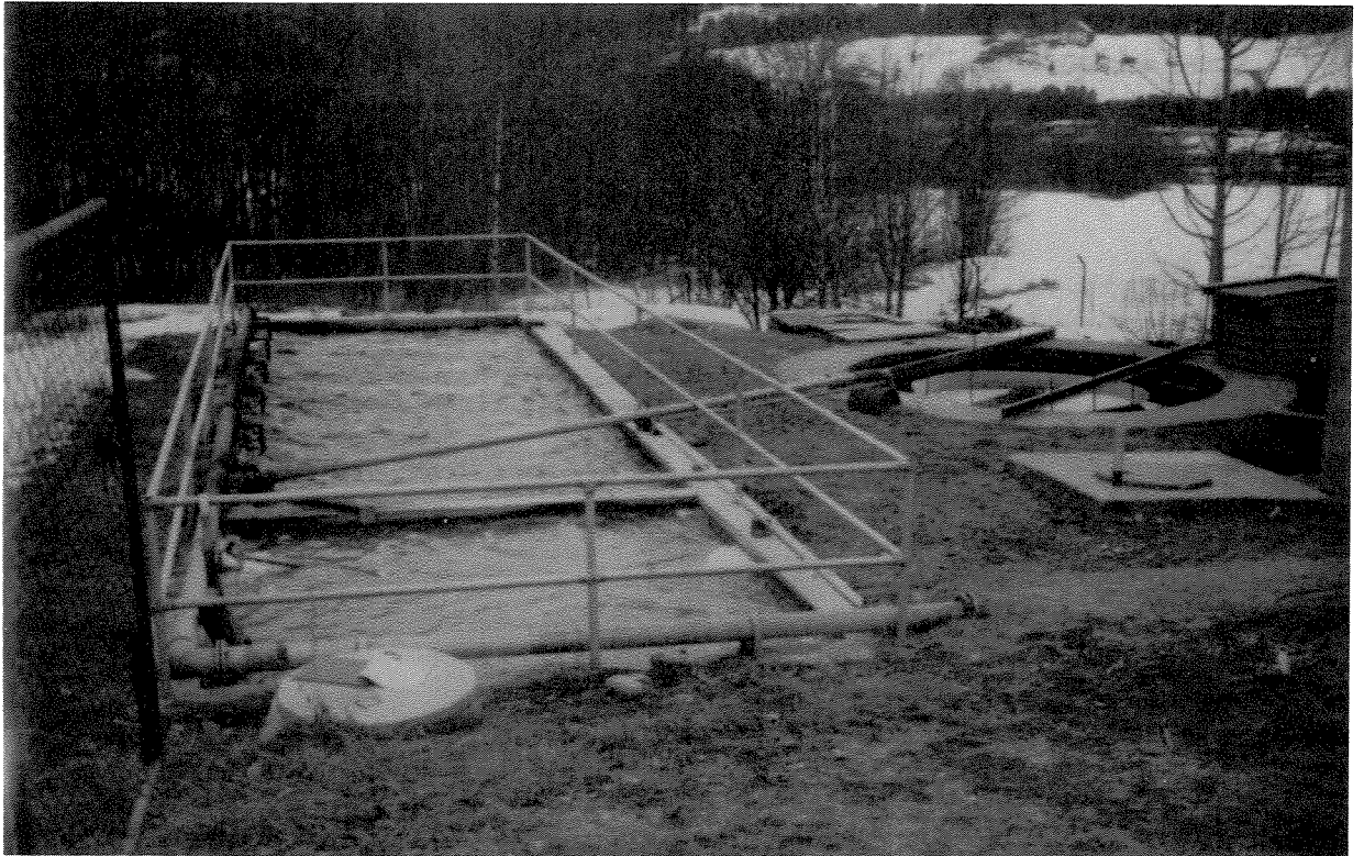
Glittre renseanlegg.
