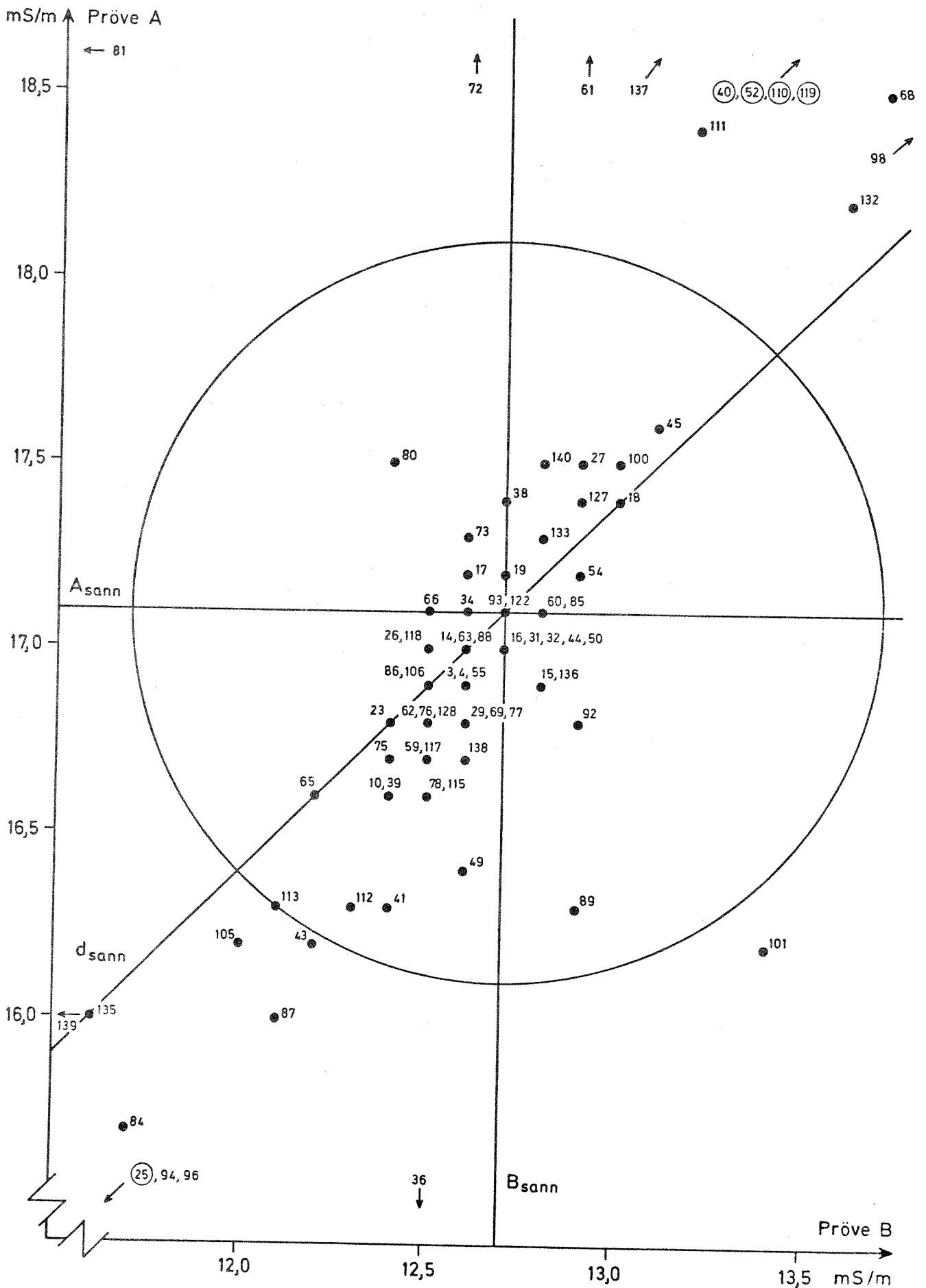
Fig.2 Konduktivitet
