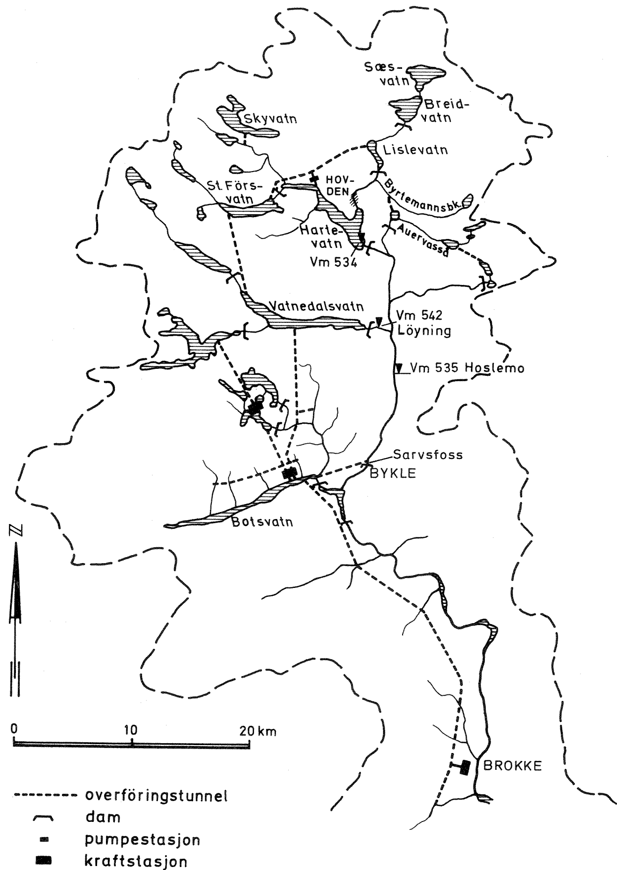
Fig. 2-1 Utførte og planlagte reguleringer etter planendringssøknad 1977
