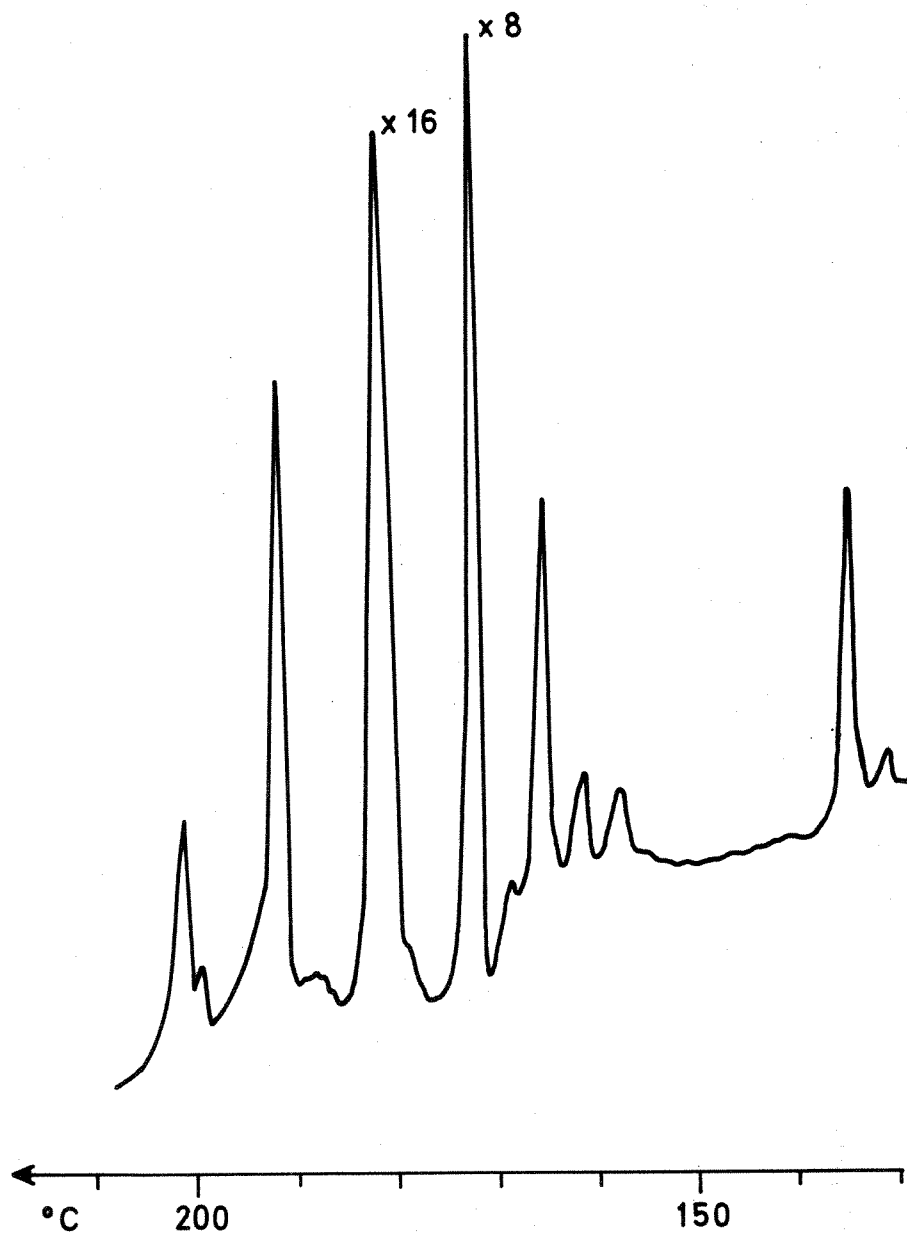
Fig. 7 Analyse av klorerte fenoler i torsk fra utløpet av Otrå
