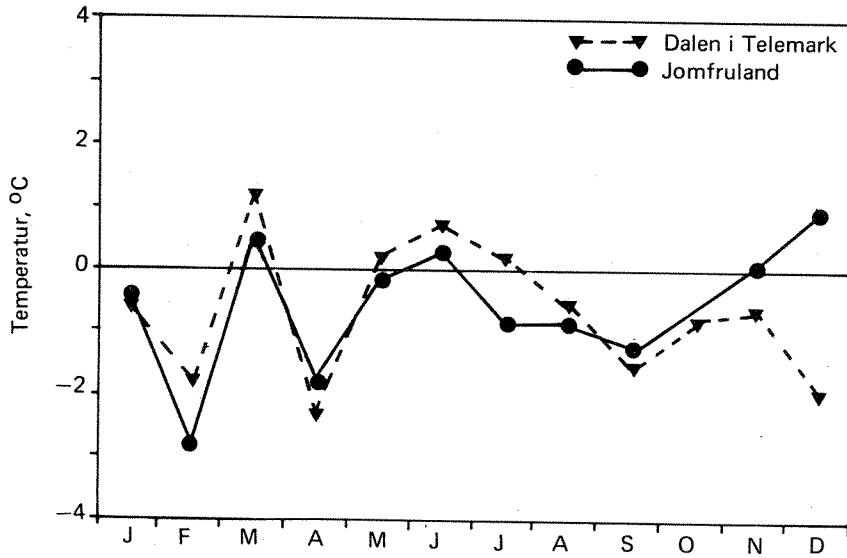
Fig. 3.4a Middelttemperaturens avvik fra normalen i 1977.
