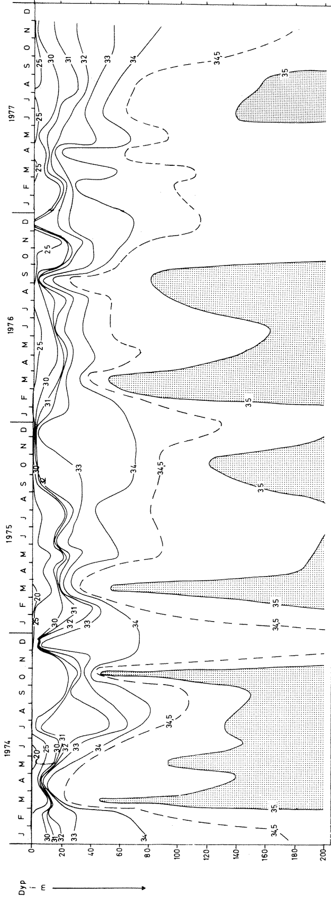
Fig. 3.9 St JH 1, Langesundbukta. Saltholdighetsvariasjoner ( ^{\circ}/_{oo} ) januar 1974 - desember 1977.
