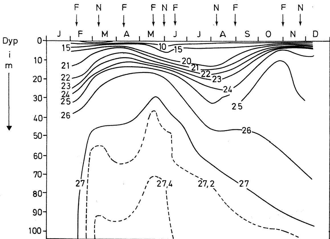
Fig. 14. St. FG-1, Brevikfjorden. Variasjoner i tetthet ( \sigma_t ) i 1978.
