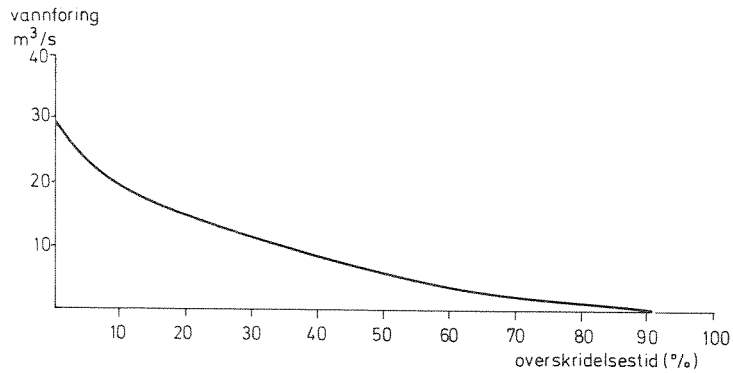
Fig 4.6.3 Nærområder til Vangsvatn Midlere årlig varighetskurver (7 døgns midler.)
