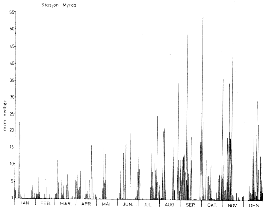
Fig. 4.7.2. Daglig nedbør og ukemiddelvanntføring. a. nedbør, Myrdal b. vannføring utløp Vangsvatnet c. nedbør, Voss
