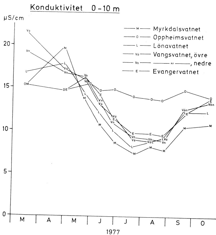
Figur 8.1.8. Konduktivitet 0 - 10 m.
