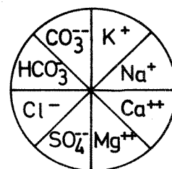
Fig. 7.1.4. Vannets innhold av de dominerende ionene (Ca, Na, K, Mg, \text{SO}_4 , \text{HCO}_3 , og \text{CO}_3 ) i noen norske innsjøer. Arealet av den stiplede sirkelen er proporsjonal med total-konsentrasjonen. Den relative konsentrasjonen av hvert ion (i % meq.) er angitt som arealet av tilhørende sirkel-sektor (se tegnforklaring nederst).
