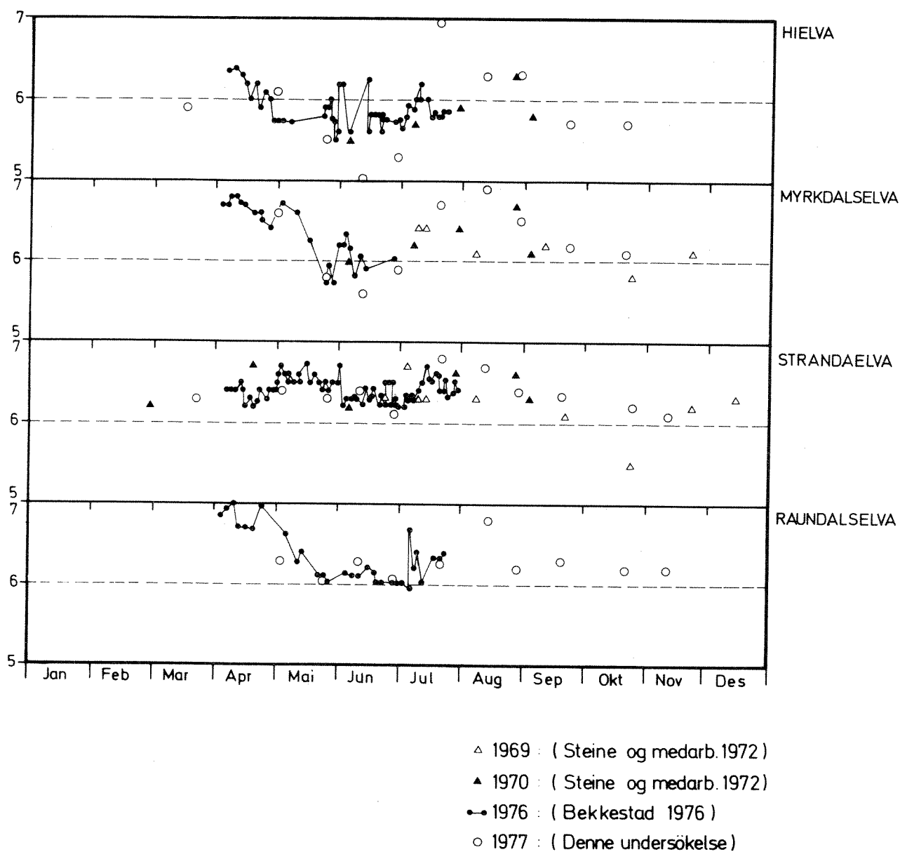
Fig. 7.1.5. pH-målinger fra fire stasjoner i Vossevatn. Stiplet strek angir pH = 6,0 for å lette sammenlikning mellom stasjonene.
