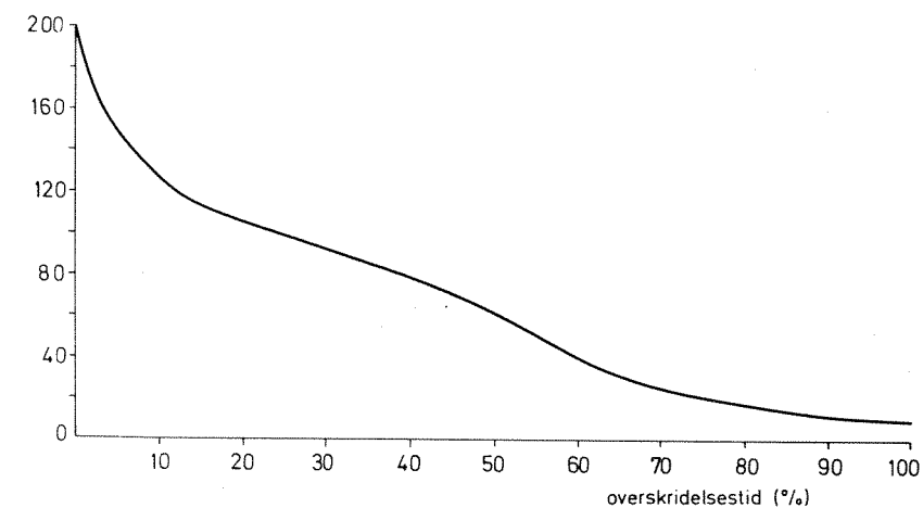
Fig 4.33 Utlöp Vangsvatn Vm 598-0 Bulken Midlere årlig varighetskurve (7 døgns midler)
