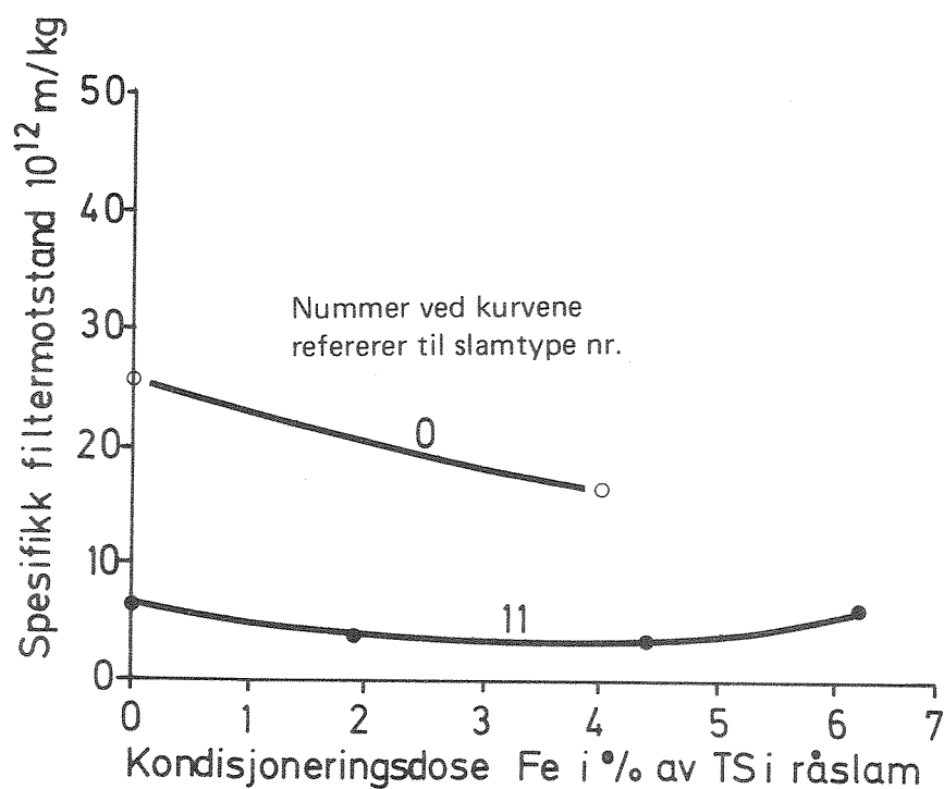
Fig. 16. Spesifikk filtermotstand ved kondisjonering med jernklorid av kalkholdige slamtyper.
