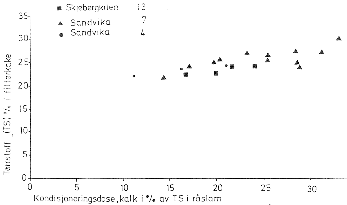
Fig. 39. Brutto TS% i filterkake for slam felt med jernklorid.
