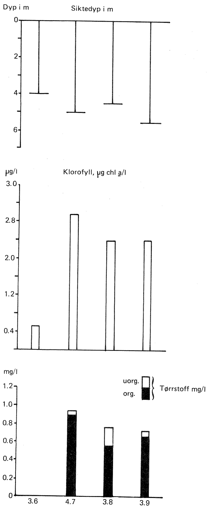
Fig. 14. Synnfjorden. Siktedyp i meter, klorofyll a ( \mu\text{g chl}_a/\text{l} ) og tørrstoff/organisk materiale (mg/l) på prøvetakingsdagene 3. juni - 3. september 1978
