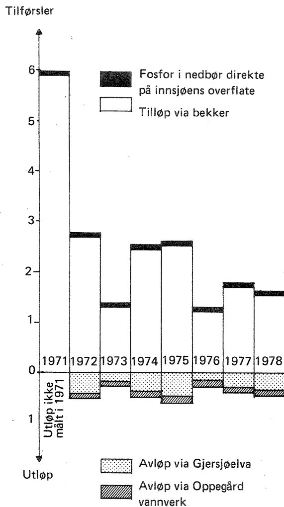
Figur 4.2.1 Fosforbudsjett for Gjersjøen (tonn fosfor pr. år).
