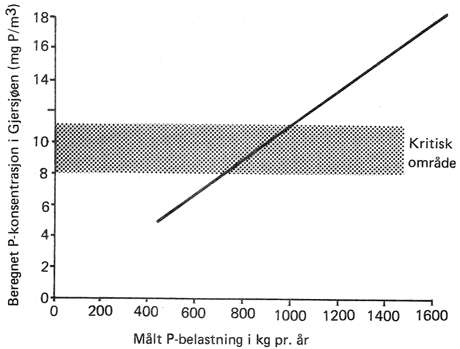
Figur 5.3.1 Beregnet fosforkonsentrasjon i Gjersjøen ved redusert fosforbelastning
