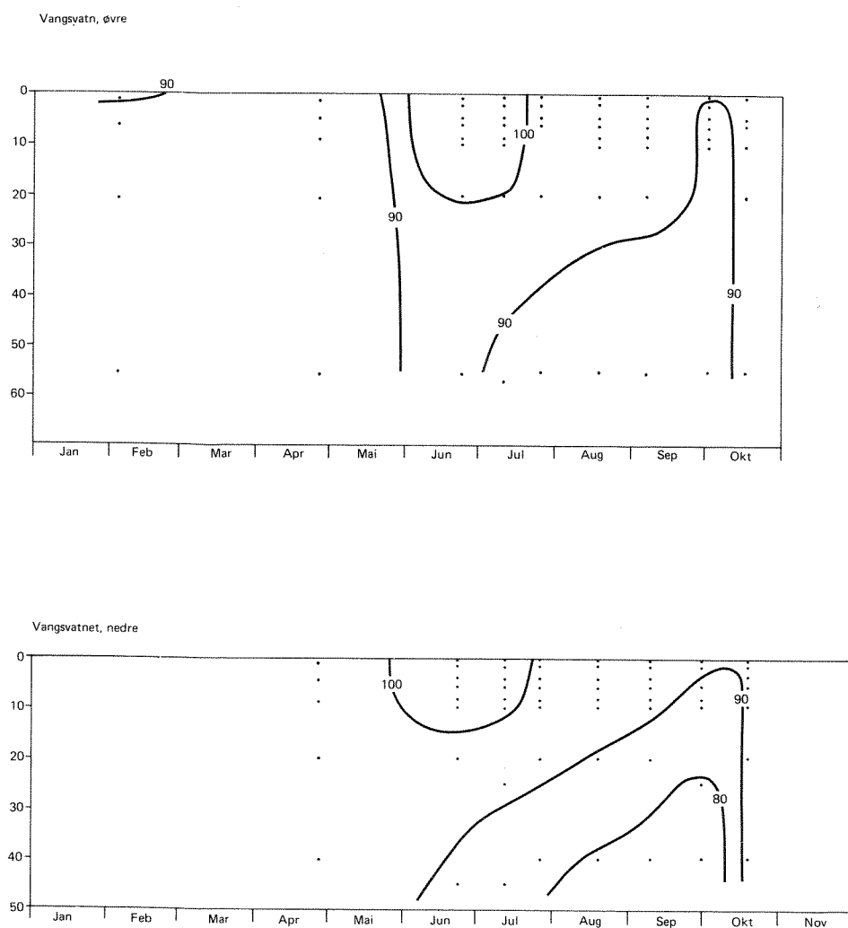
Fig. 4.5 Vangsvatnet. Oksygenmetning 1978
