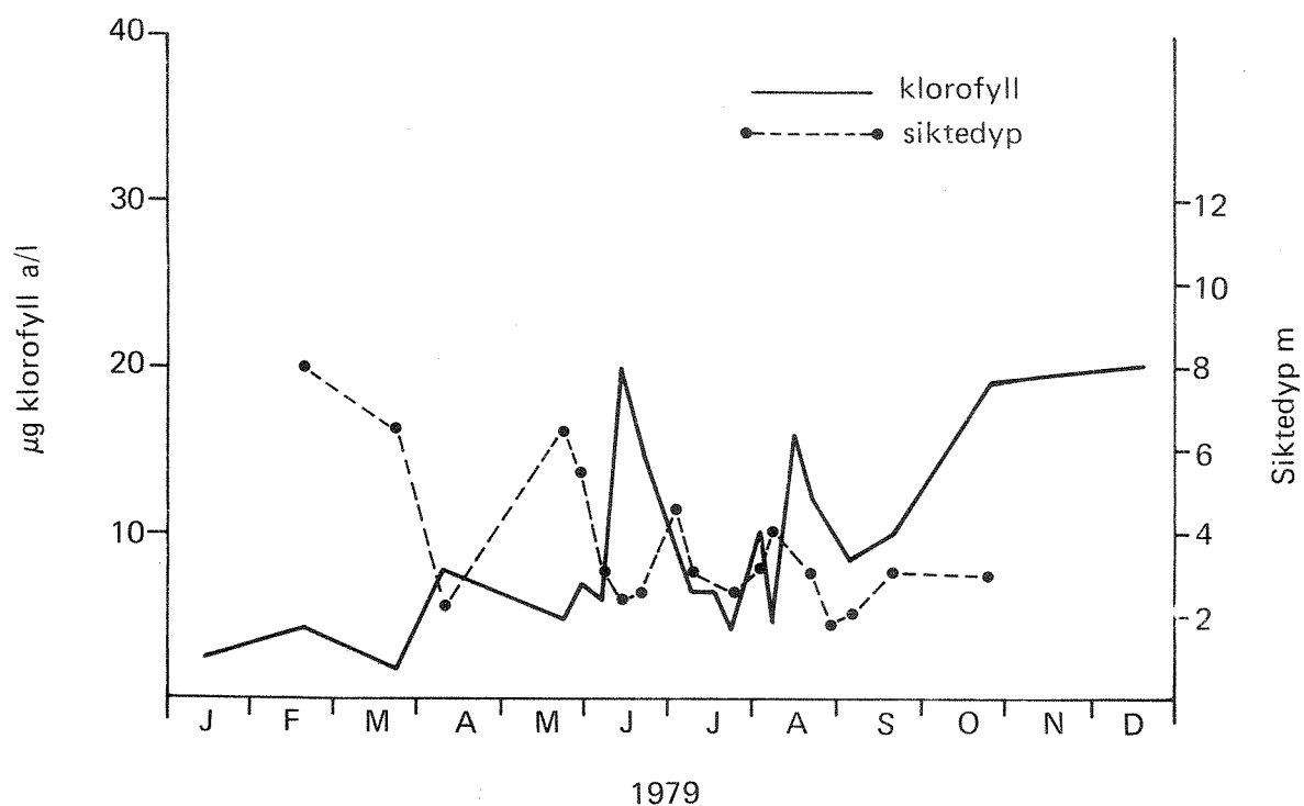
Fig. 19. Klorofyll a i 0-2 meters dyp og siktedyb i Bunnefjorden (EP1) 1979.
