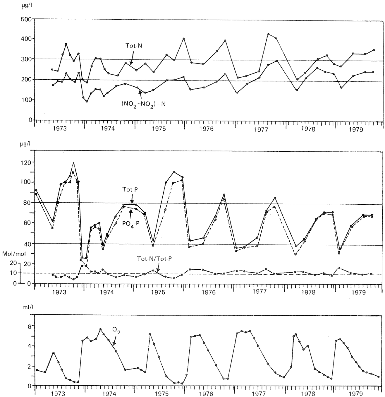
Fig. 18. Variasjonen av total nitrogen, nitrat og nitritt, total fosfor, ortofosfat ( \mu\text{g/l} ) og forholdet total nitrogen / total fosfor ( \text{mol/mol} ), samt oksygeninnholdet ( \text{ml/l} ) i Vestfjorden (DK1) på 80 meters dyp 1973-79.
