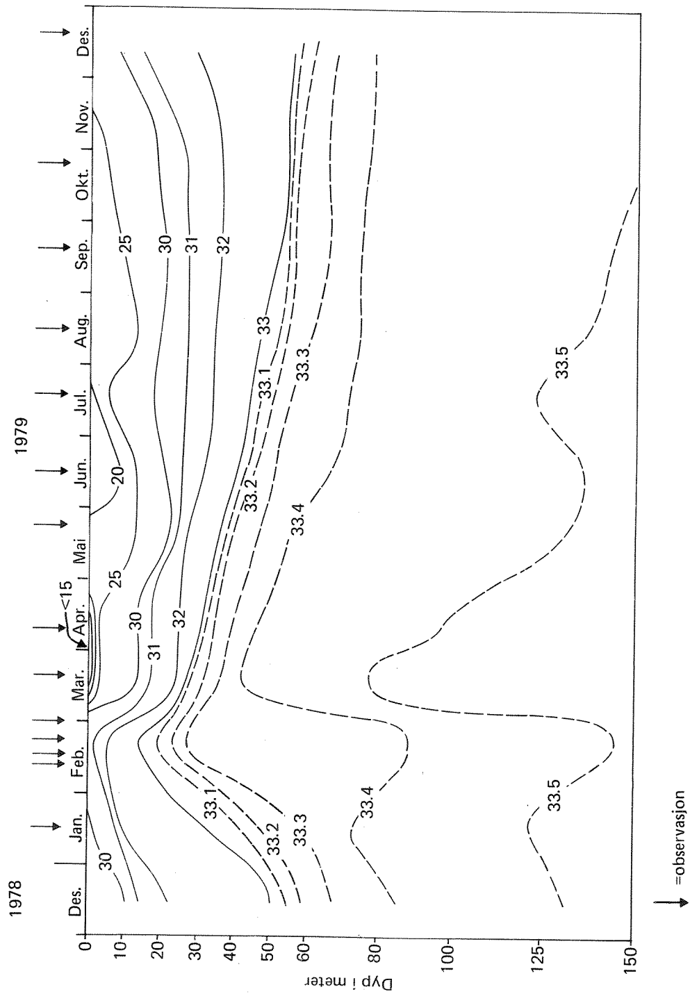
Fig. 10. Saltholdighetsvariasjonen (‰/oo) i Bunnefjorden (EPI) 1979.
