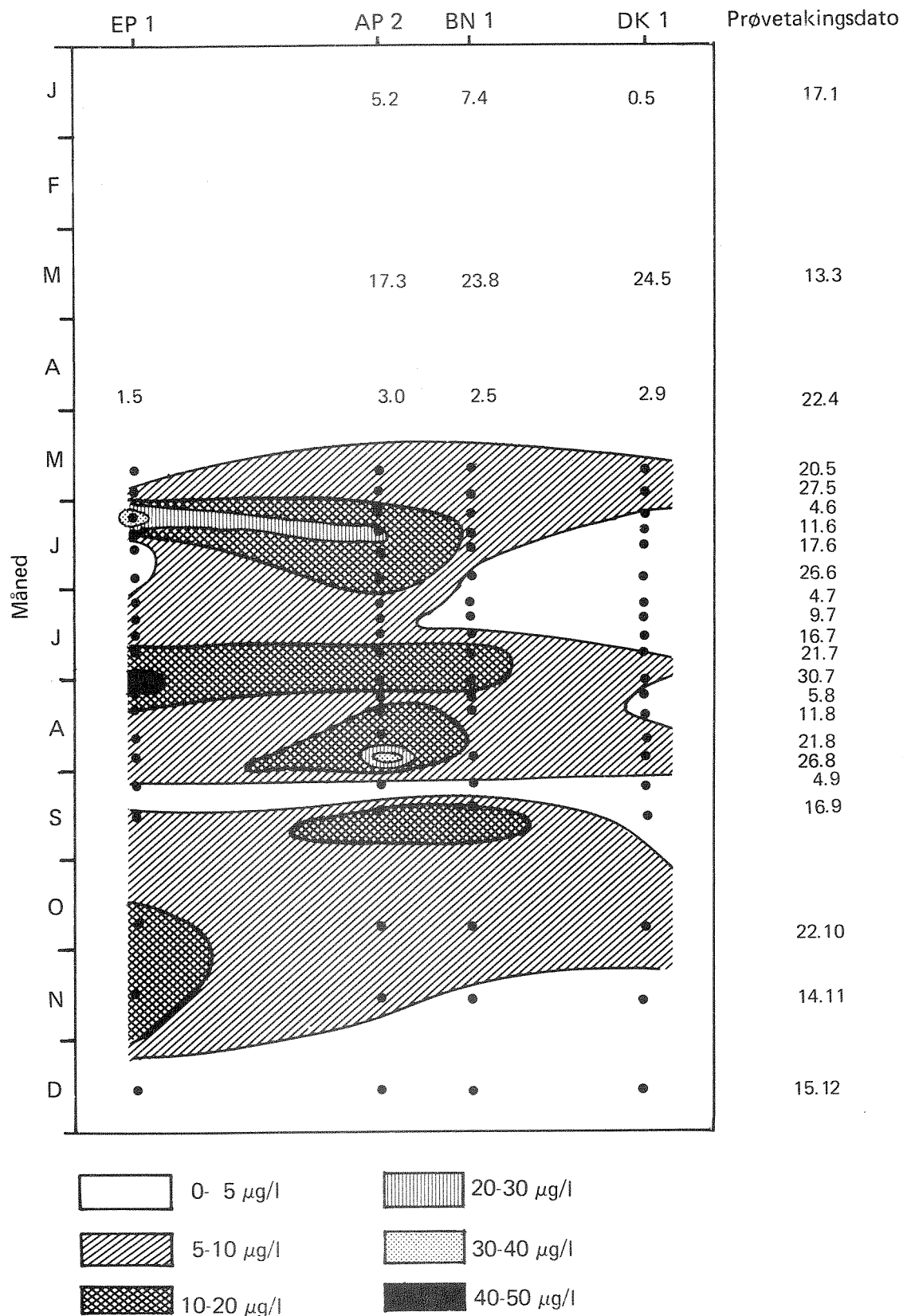
Fig. 31. Klorofyll a i 0-2 meters dyp fremstilt som variasjon over tid for fire stasjoner i indre Oslofjord 1980.
