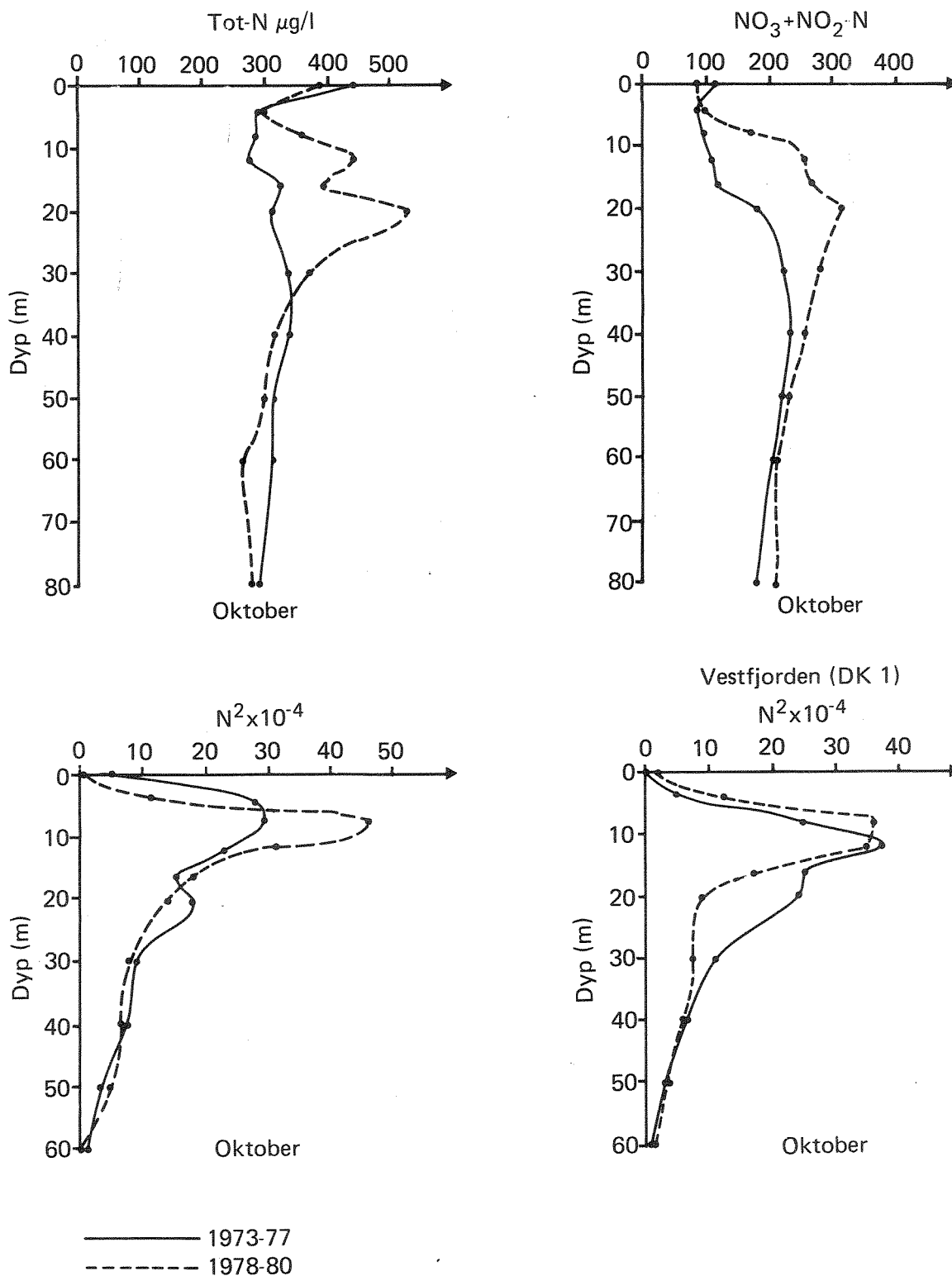
Fig. 26. Middelerdi av total-nitrogen, nitritt og nitrat, samt vannets stabilitet ved Vasilää-Brunt frekvensen i Lysakerfjorden (BN1) 1973-77 og 78-80, samt for Vestfjorden i oktober måned.
