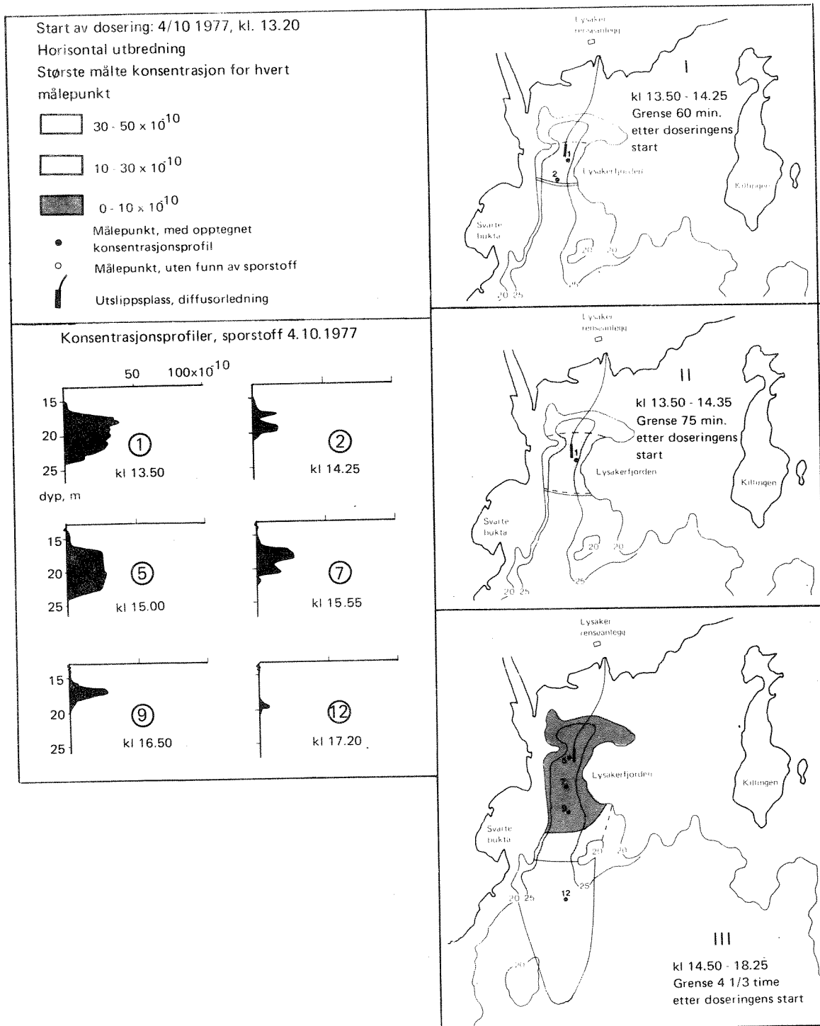
Fig. 24. Spredning av sporstoffmerket avløpsvann fra Lysaker Renseanlegg i Lysakerfjorden.
