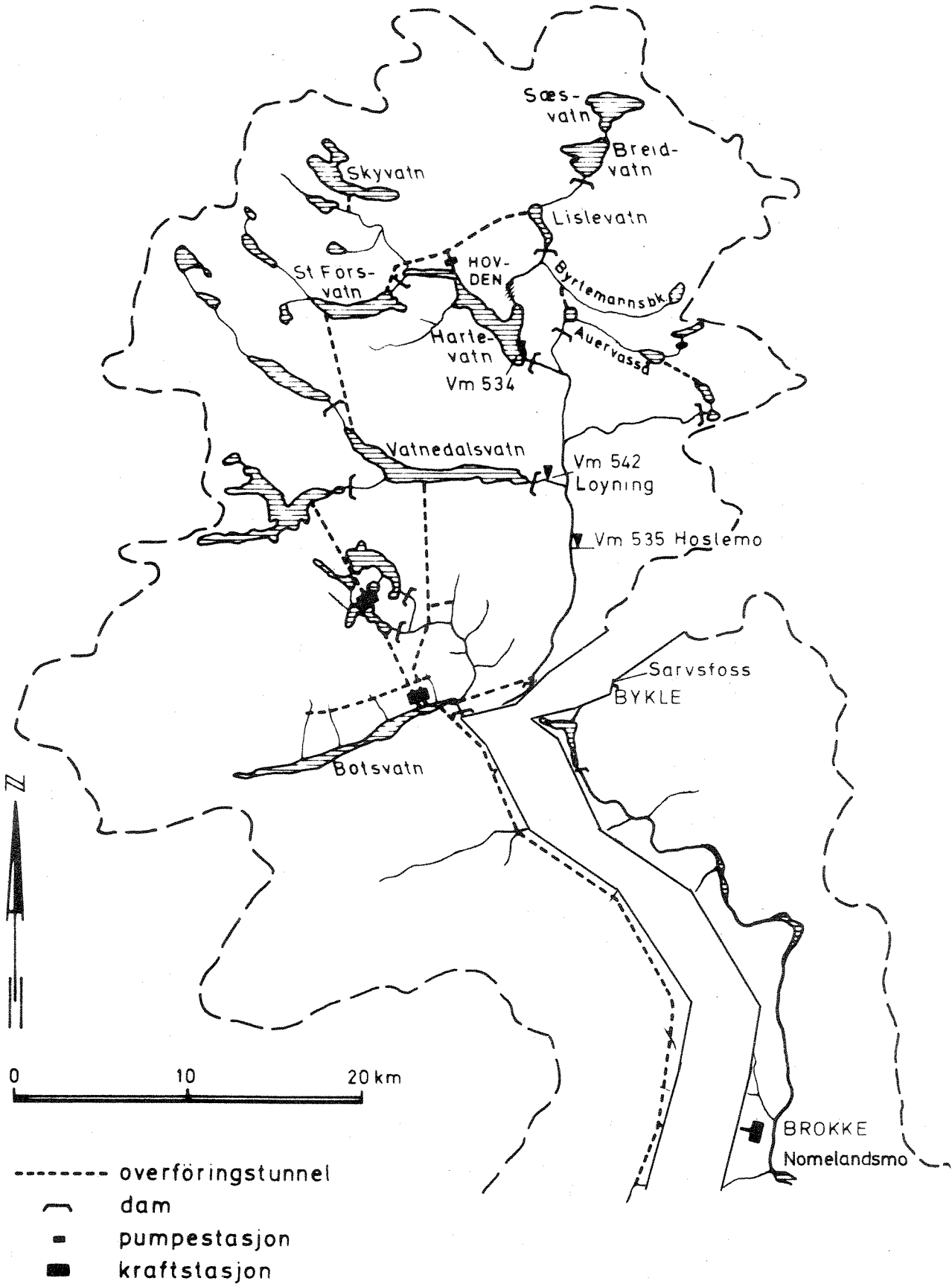
Fig. 10. Reelt nedbørfelt etter full utbygging.
