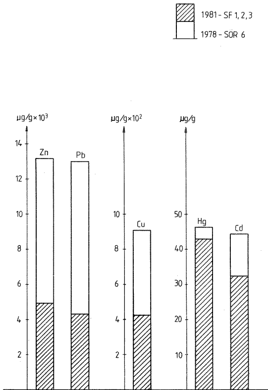
Fig. 10. Sammenligning av innholdet (µg/g ts) av sink (Zn), bly (Pb), kopper (Cu), kvikksølv (Hg) og kadmium (Cd) i sedimentene i Odda havnebasseng i 1981 (gj.sn. SF1, 2, 3, 0-1 cm) med verdiene fra 1978 (SØR 6, 0-2 cm).
