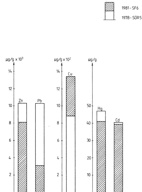
Fig. 11. Sammenligning av innholdet (µg/g ts) av sink (Zn), bly (PB), kopper (Cu), kvikksølv (Hg) og kadmium (Cd) i sedimentene ved Tyssedal i 1981 (SF 6, 0-1 cm) med verdiene fra 1978 (SØR 5, 0-1 cm).
