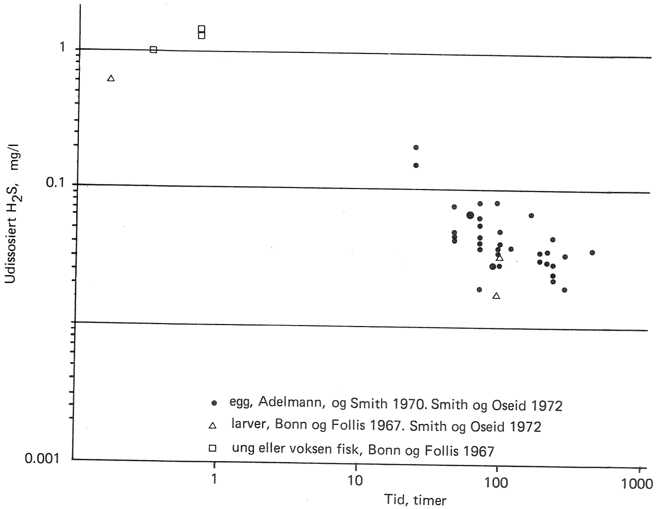
Figur 12. Sammenheng mellom letal konsentrasjon av udissosiert hydrogensulfid og eksponeringstid for fisk.
