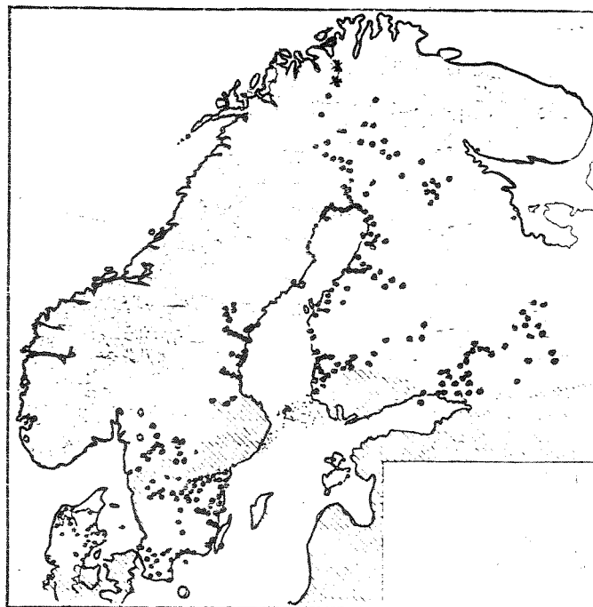
Fig. 7.2. Utbredelse av Butomus umbellatus i Norden . Etter Hulten, * Altavassdraget 1981
