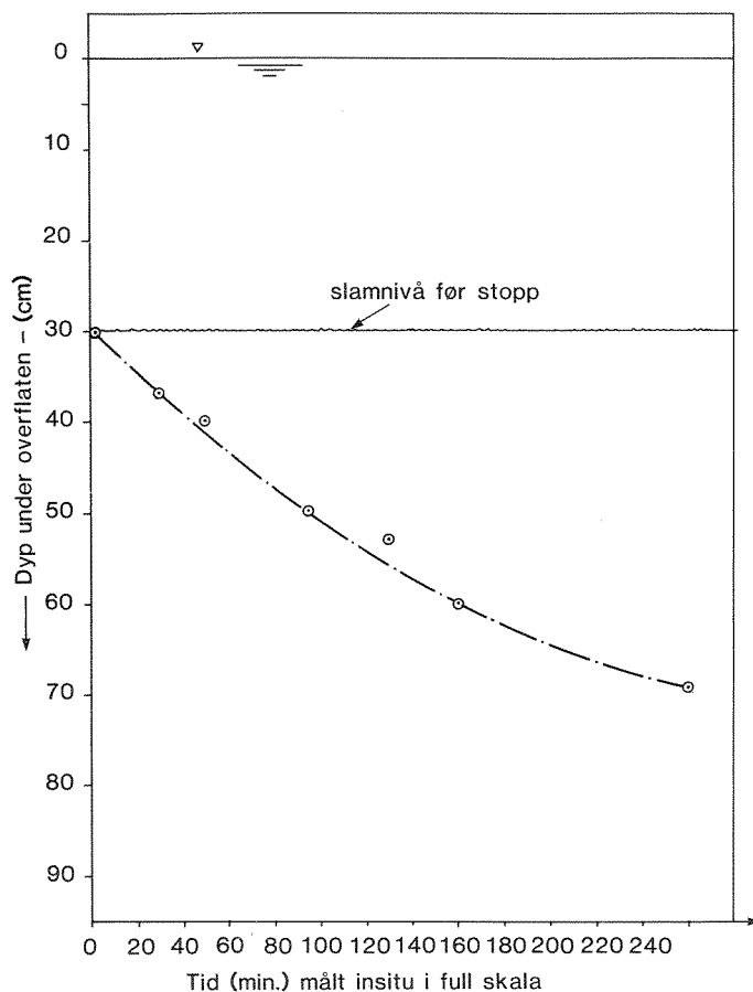
Figur 21. Undersøkelse av slamteppenivåsenkning i forsøkslinjens sedimenteringsbasseng målt i in situ i fullskala 27.5.81 ved HIAS
