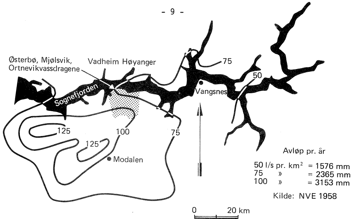
Fig. 2-2. Arlige middelavløp i de regulerte vassdragene er stort sett høyere enn 75 l/s pr km 2 ≈ 2300 mm.
