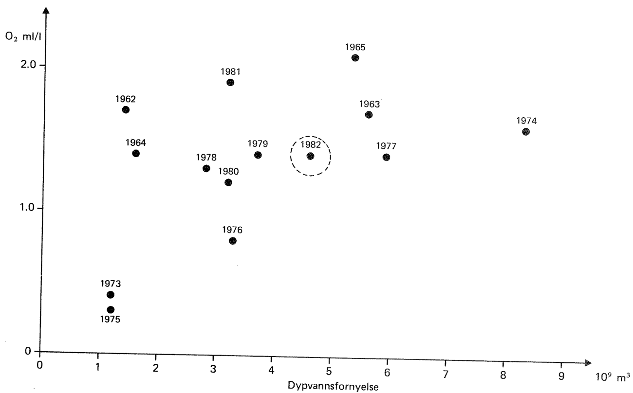
Fig. 16. Dypvannsfornyelse og oksygenkonsentrasjonen (oktober måned) på 80 meters dyp i Vestfjorden (DK1) 1962-65 og 1973-82
