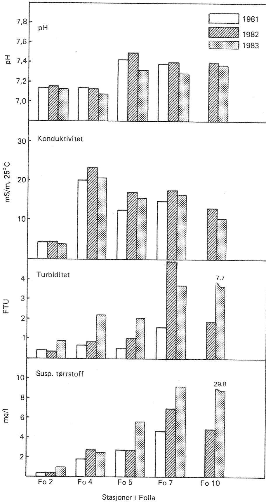
Fig. 5. Kjemiske analyseresultater for Folla. Middelerverdier 1981-83.
