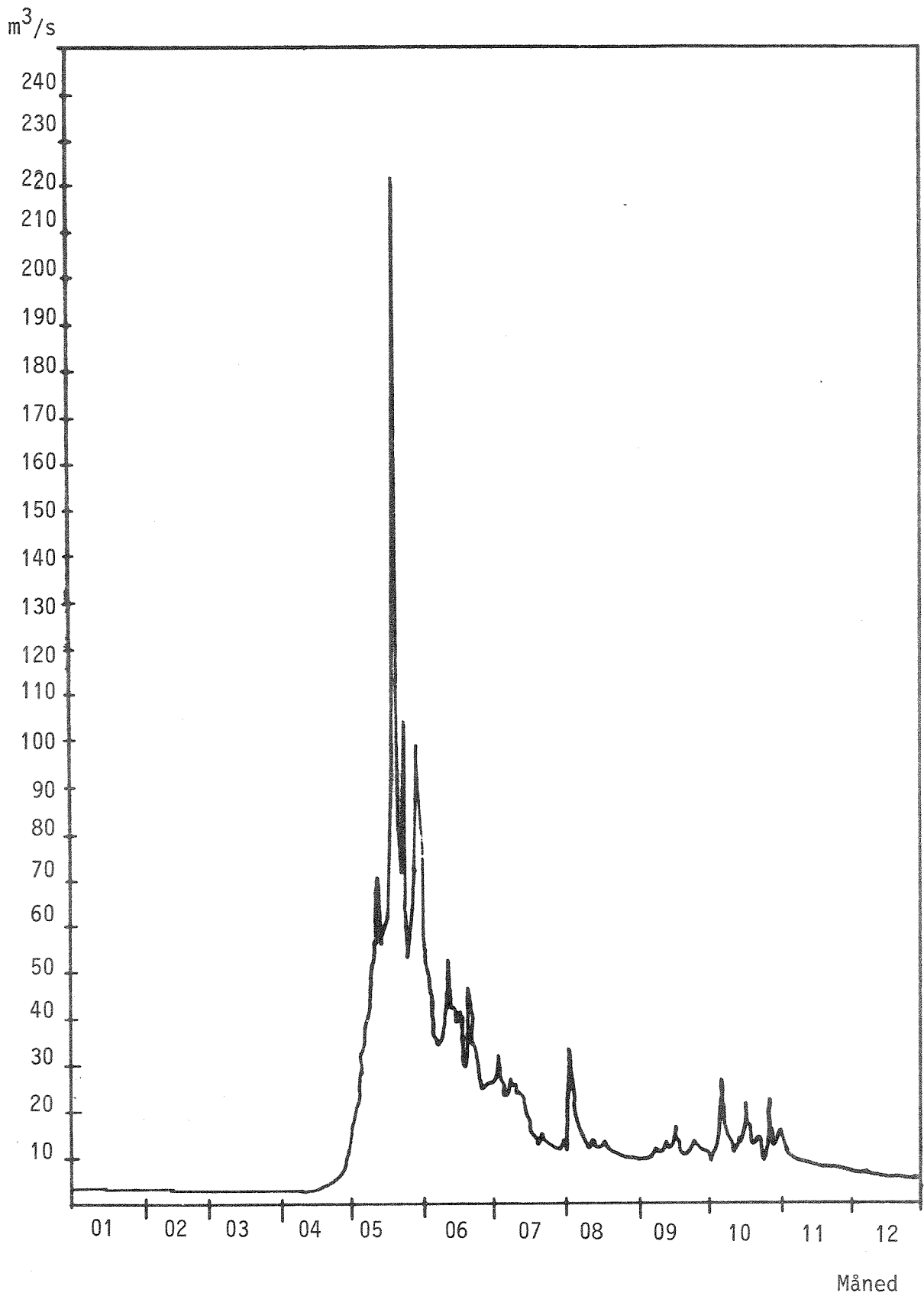
Fig. 4. Vannføringen i Folla ved Ryfetten 1983.
