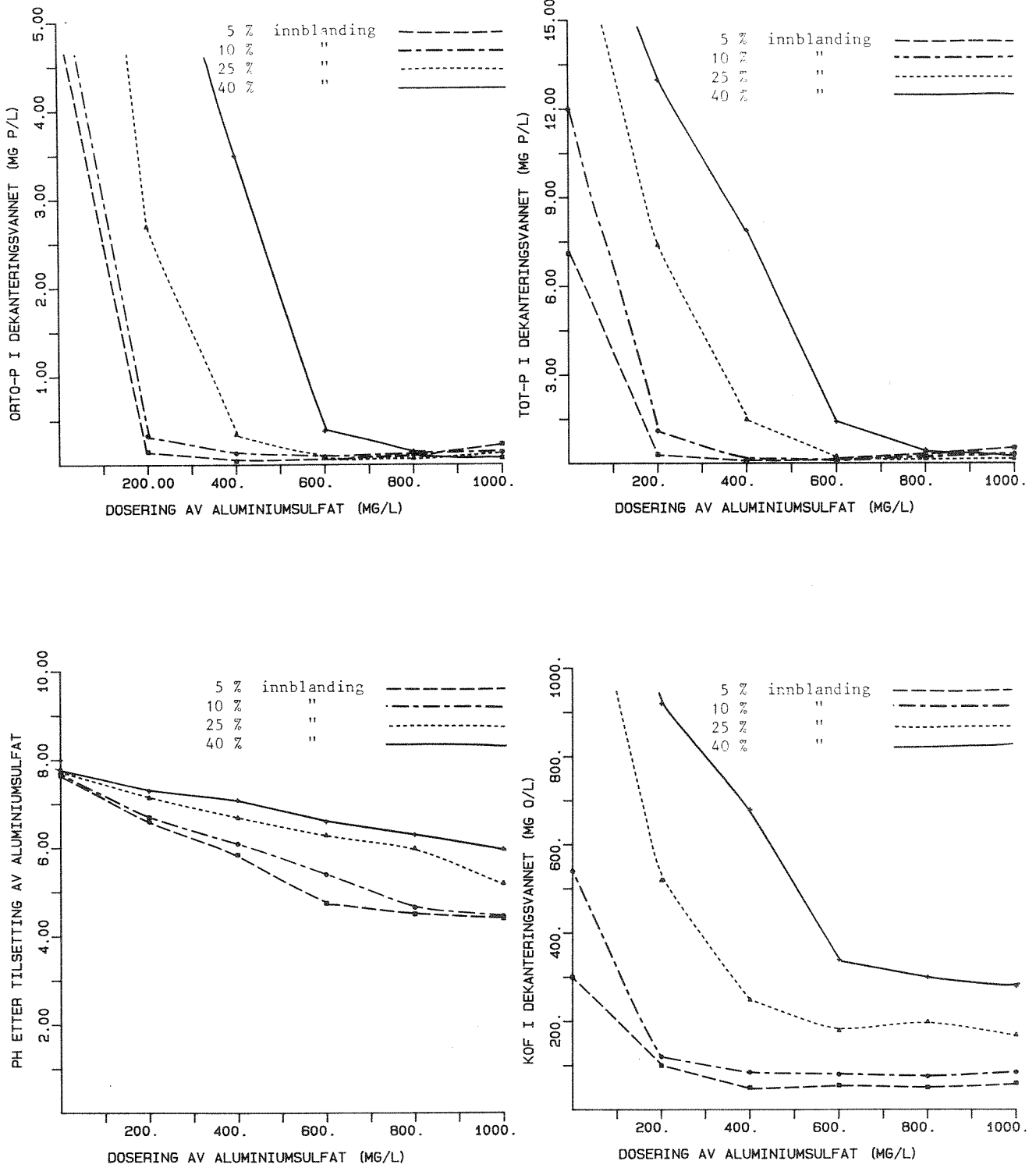
Figur 4.1. Orto-P, Tot-P, pH og KOF som funksjon av dosering, Jar-test med tilsetning av ubehandlet slamvann.
