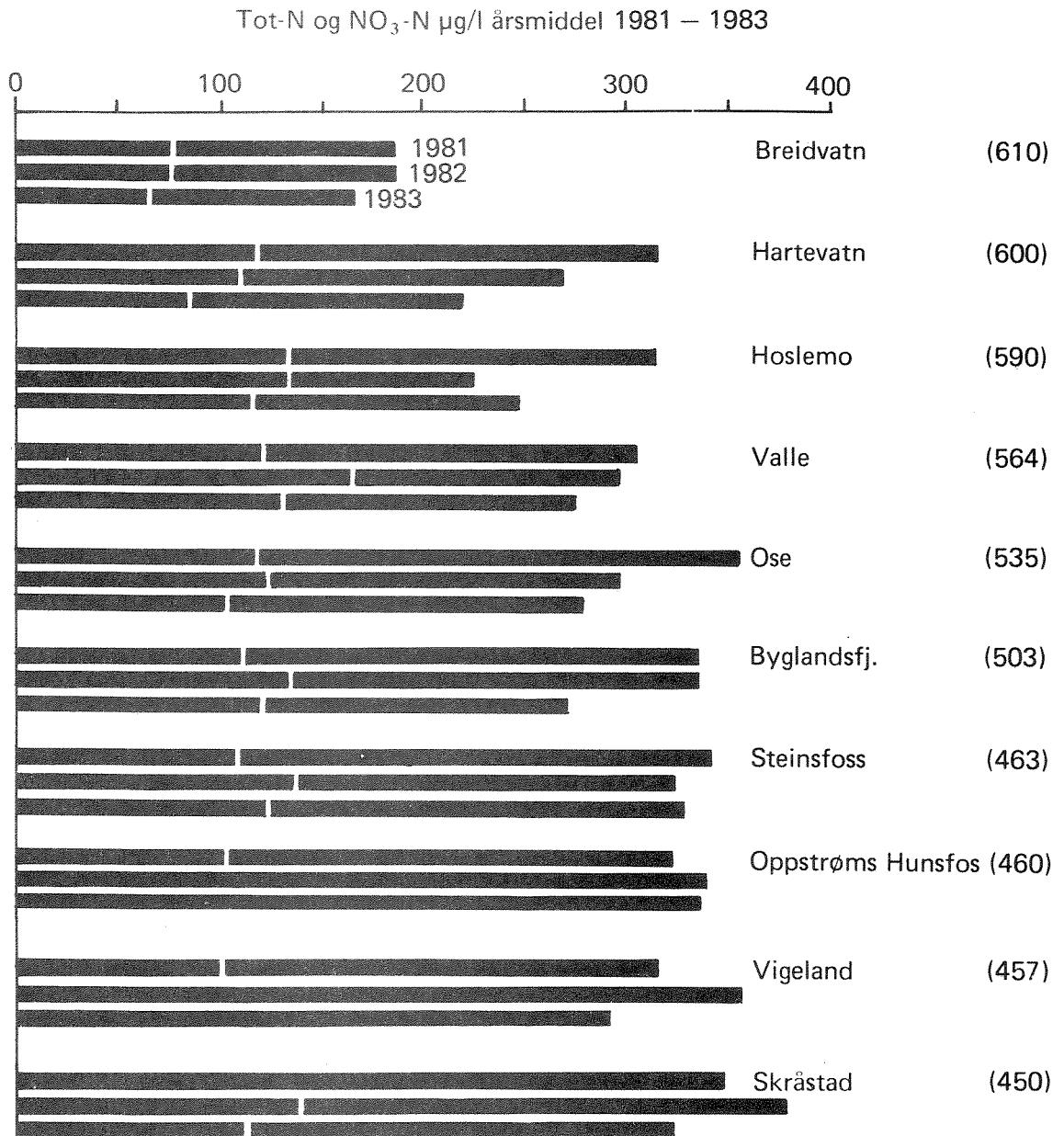
Figur 6. Årsmiddelkonsentrasjon av total-nitrogen (hele søylen) og nitrat-nitrogen (nedre del av søylen) i 1981, 1982 og 1983 i rutineprøver fra Otra.
