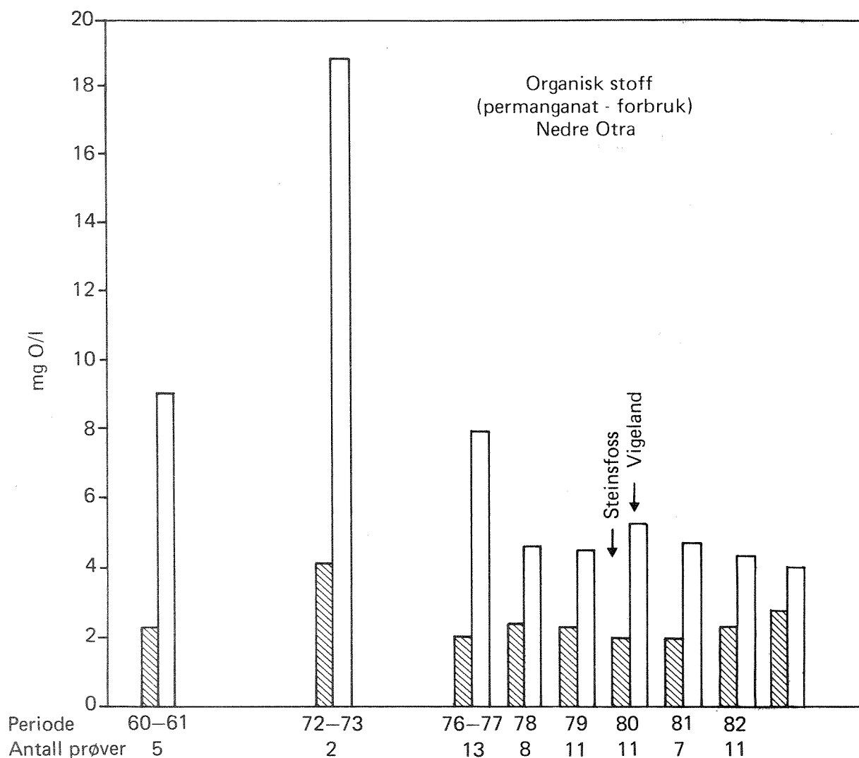
Figur 10. Middelkonsentrasjon av organisk stoff (målt som permanganatforbruk, mg O/l) ved Steinsfoss ovenfor og Vigeland nedenfor industriutslippene ved Vennesla. Siden 1977 har økningen i konsentrasjon blitt mindre som følge av rensetiltak ved fabrikkene. Utslippene er imidlertid fremdeles store nok til å gi en 50 % økning i konsentrasjonen av organisk stoff i elva.
