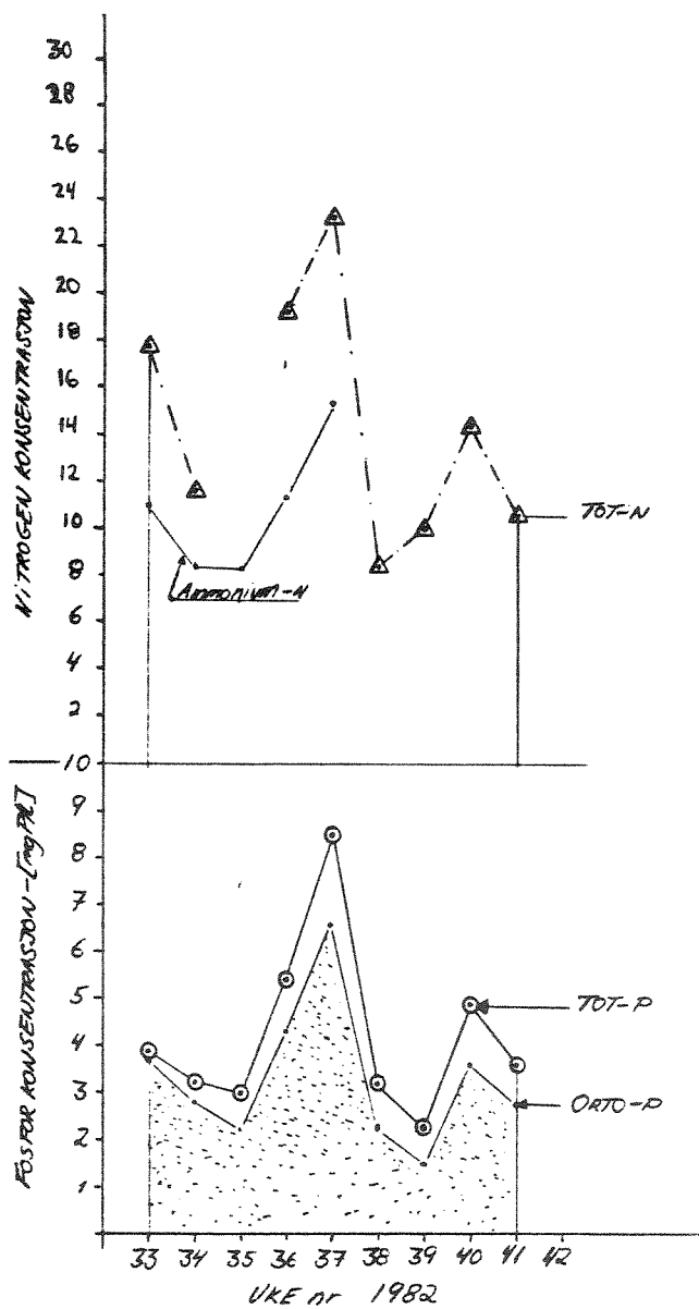
Figur 3. Analysekonentrasjoner av fosfor, ortofosfat, Tot-N og ammonium i innløpsvannet til Buhrestua rensanlegg høsten 1982.
