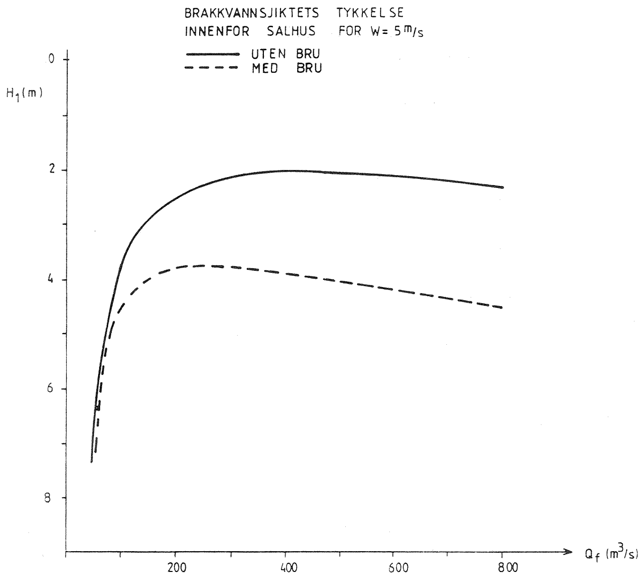
Fig. 4.17. Brakkvannslagetets tykkelse innenfor Salhus med og uten bro for en blandingsvind W = 5 \text{ m/s} (etter Gjerp m.fl. 1982).
