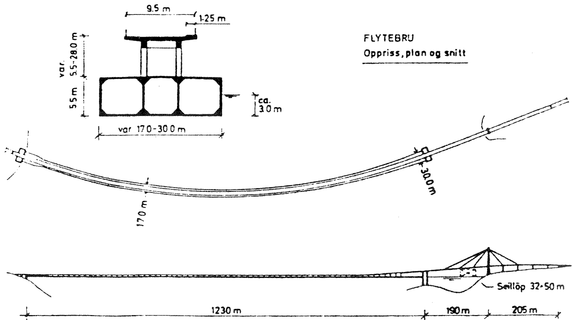
Fig. 2.1. Flytebro over Salhusfjorden. (Etter St.meld. nr. 75 - 1979-80).
