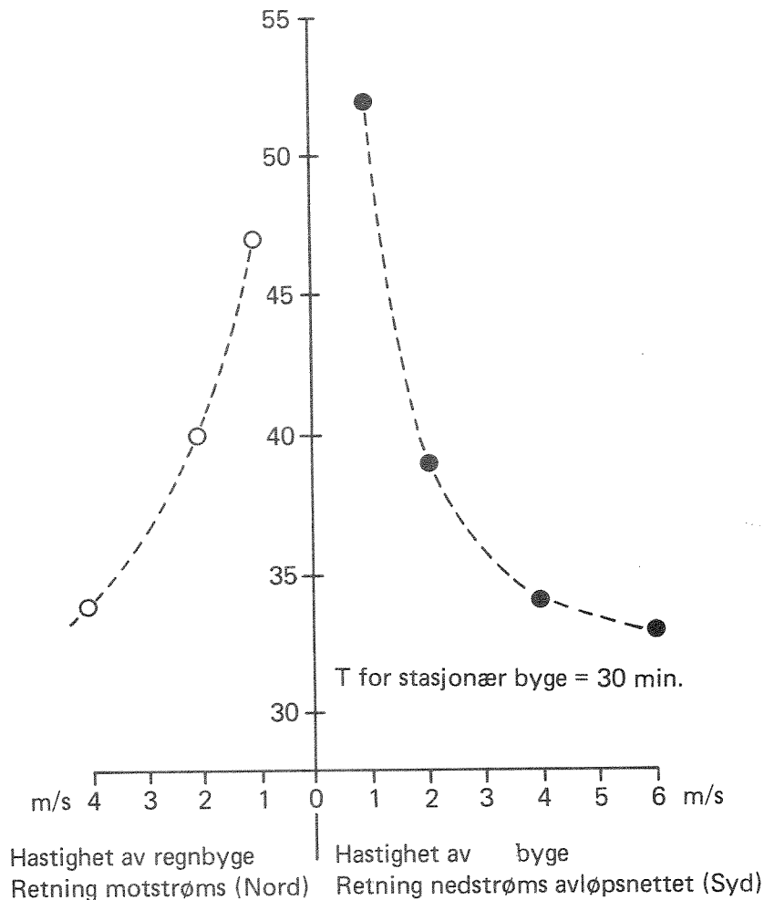
Figur 5.4. Tidspunkt for maksimalavrenning ( Q_{maks} ) fra Søren Jaabæks gate ved varierende hastighet for regnbyge. Regnskyll er to-års regnet fra Blindern som hyetogram.
