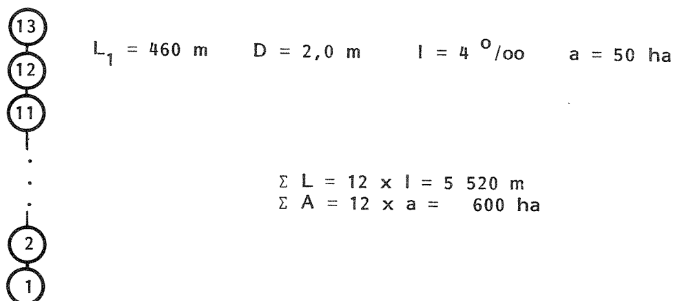
Figur 4.3. Hypotetisk avløpsfelt.
