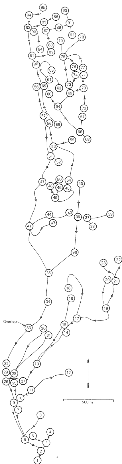
Figur 4.2. Avløpsnett i Lilleaker feltet.
