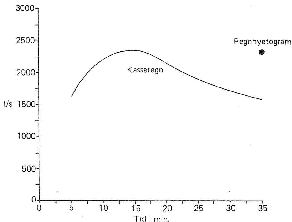
Figur 6.14. "Avlangt" felt. Q_{maks} for 2-års regnhyetogram og for 2-års kasseregn.
