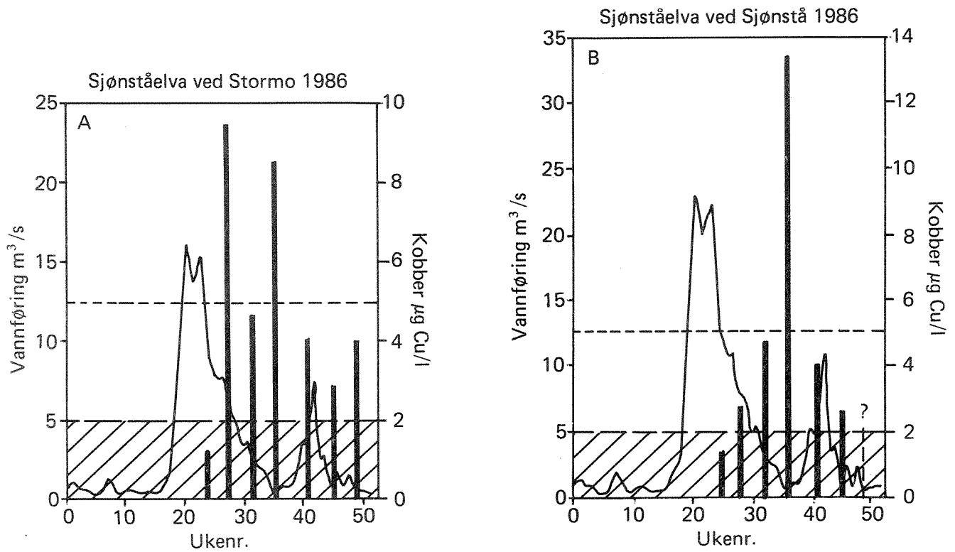
Figur 7. Sjønståelva ved Stormo (A) og Sjønstå (B) 1986. Vannføring (heltrukken linje) og kobberkonsentrasjon. EIFACs grenseverdi for kobber (5µg Cu/l, 95-prosentil) er stiplet.
