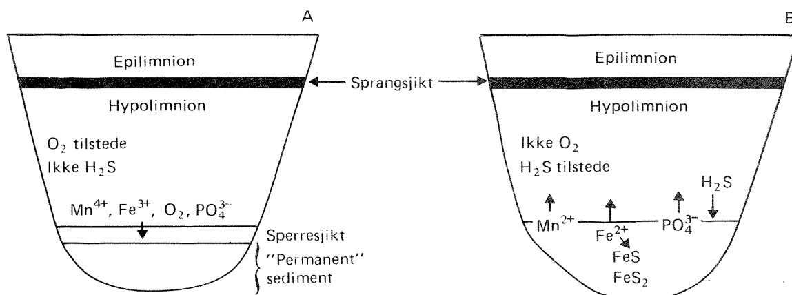
Figur 4.2 Sedimentenes innvirkning på vannkvaliteten. Mobilisering av fosfatfosfor ( PO_4^{3-} ), jern ( Fe^{2+} ) og mangan ( Mn^{2+} ) som følge av at oksygenet er brukt opp ved nedbryting av organisk stoff (alger). Ved tilstrekkelig oksygen i vannet (A), er det etablert et sperresjikt i sedimentoverflaten hvor mangan og jern binder bl.a. fosfater. Disse forbindelser er praktisk talt uløselig i oksygenholdig vann. Når oksygenet blir borte (B), reduseres mangan og jernforbindelsene og går derved over til en lett løselig form. Resultatet blir høyt innhold av mangan, jern og fosfater i det oksygenfrie vannet. Er hydrogensulfid til stede i vannet vil jernet binde seg med sulfidene og falle ut som tungt løselig jernsulfid.
