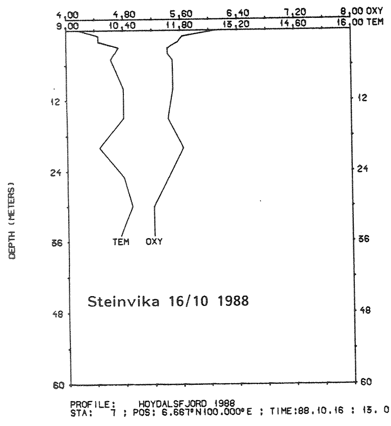
Fig. 4.1.e-g. Vertikalprofilar av Salinitet (SAL), temperatur (TEM), oksygen (OXY) og densitet (SGM) i Høydalsfjorden i perioden september-oktober 1988.
