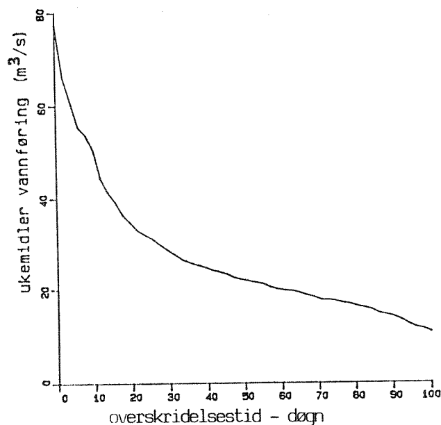
Fig. 7. Midlere årlig varighetskurve for Sjonstaelva ved Fjell på bakgrunn av data fra perioden 1970-83.
