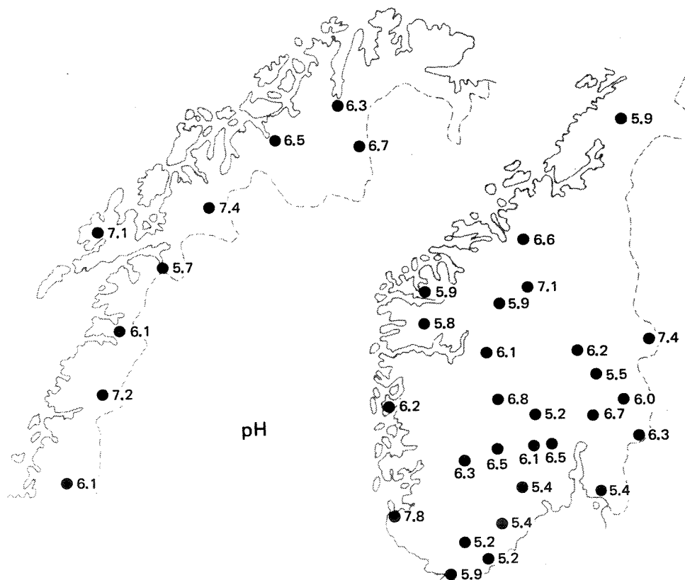
Fig. 10. Landsomfattende grunnvannnett (LGN) - Middelerverdier for pH for perioden 1981-1987.
