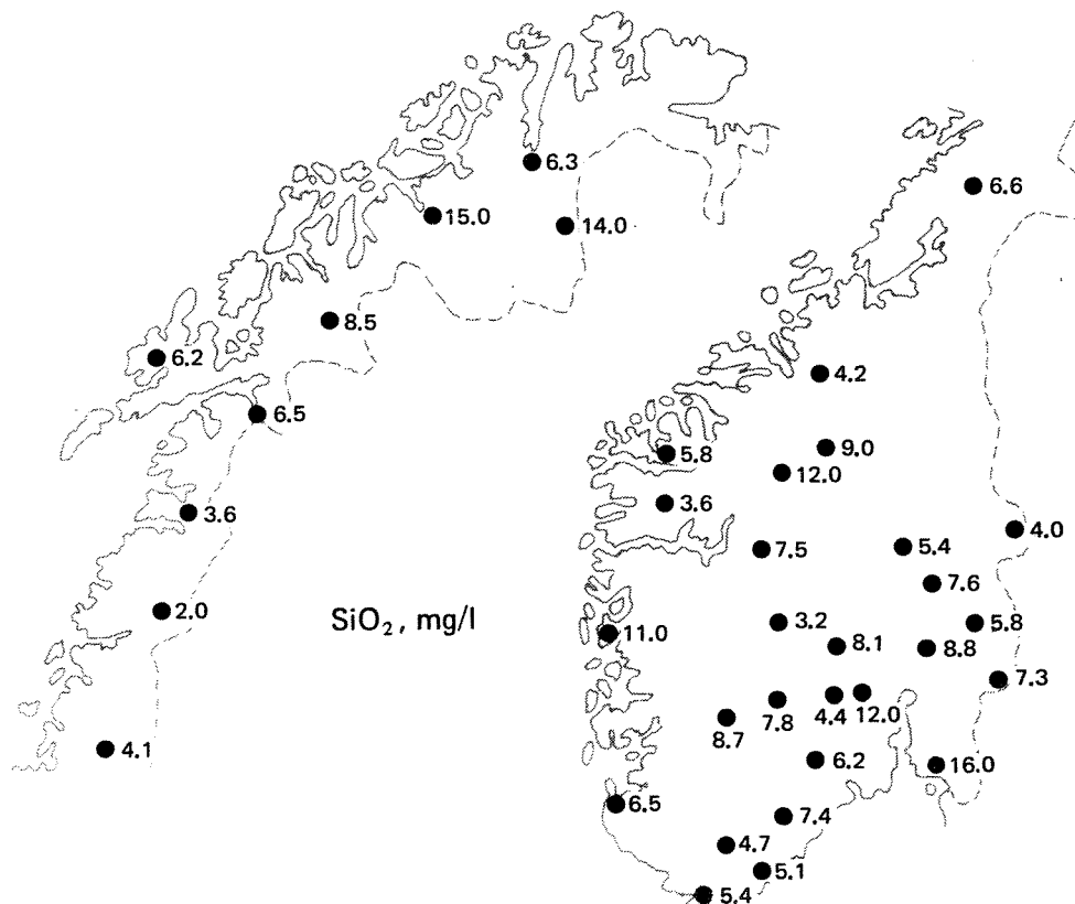
Fig. 11. Landsomfattende grunnvannnett (LGN). - Middelerverdier av silisium for perioden 1981-1987.
