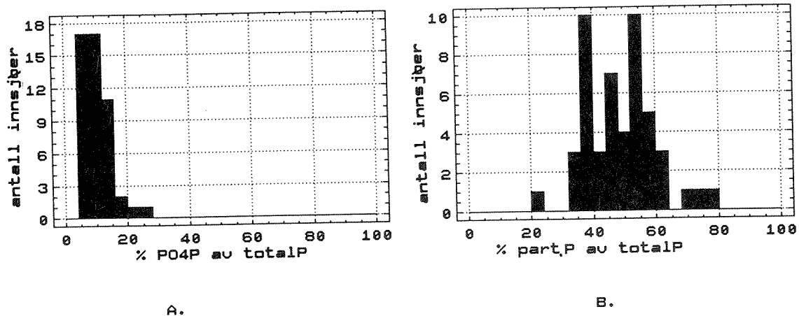
Figur 4.2.7 Andel fosfat (A.) og partikulært P (B.) av totalfosfor i 1989 (sesongmiddelverdier)
