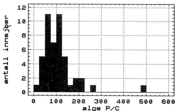
Figur 5.2.1 Algenes P/C-forhold beregnet fra middelveier for 1989
