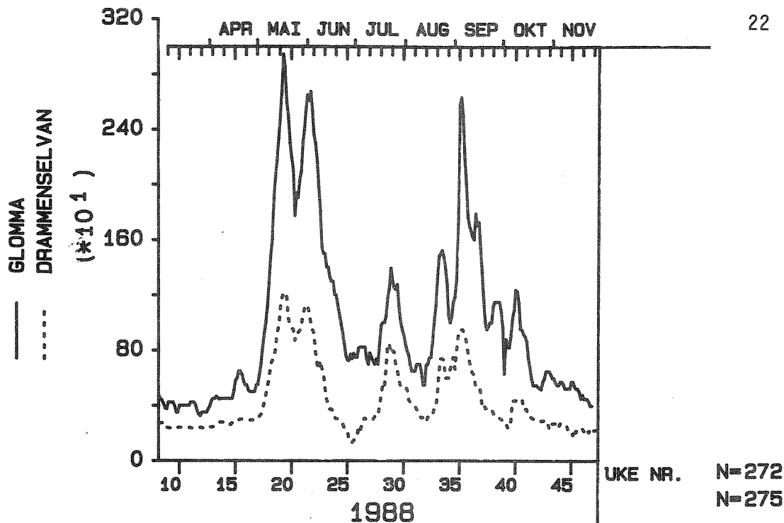
Figur 5. Vannføringen (m 3 /s) i Glomma og Drammenselva 1988.
