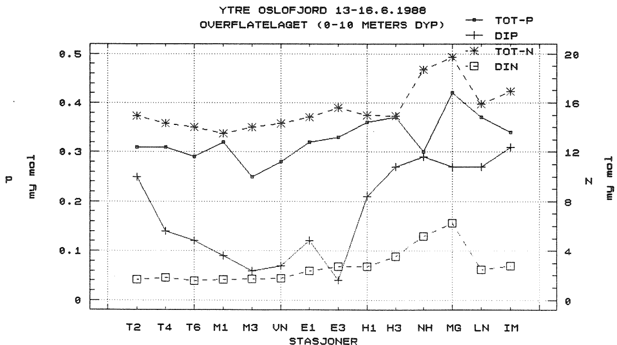
Figur 15. Overflatelagets nærings盐konsentrasjon ( \mu\text{M} ) som gjennomsnitt av observasjoner fra 0-10 meters dyp i juni 1988.
