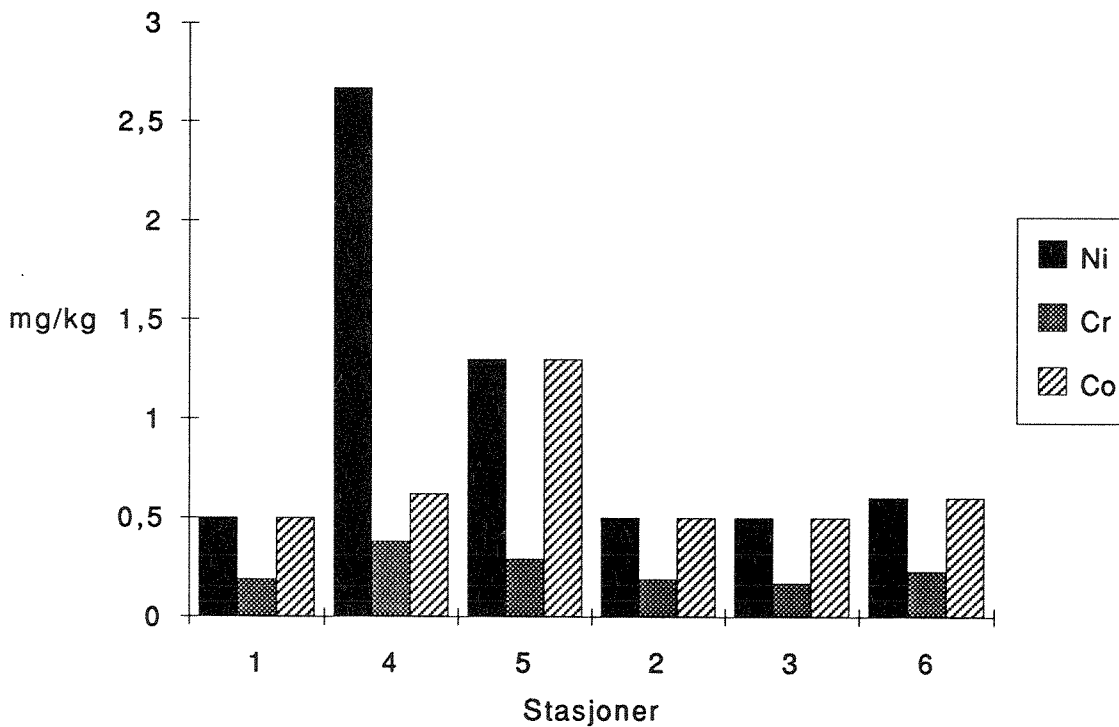
Figur 28. Innholdet av sink, kobber, bly, nikkel, krom og kobolt i grisetang fra Ballangfjorden 1989. (Konsentrasjonene er beregnet på tørrvektsbasis).
